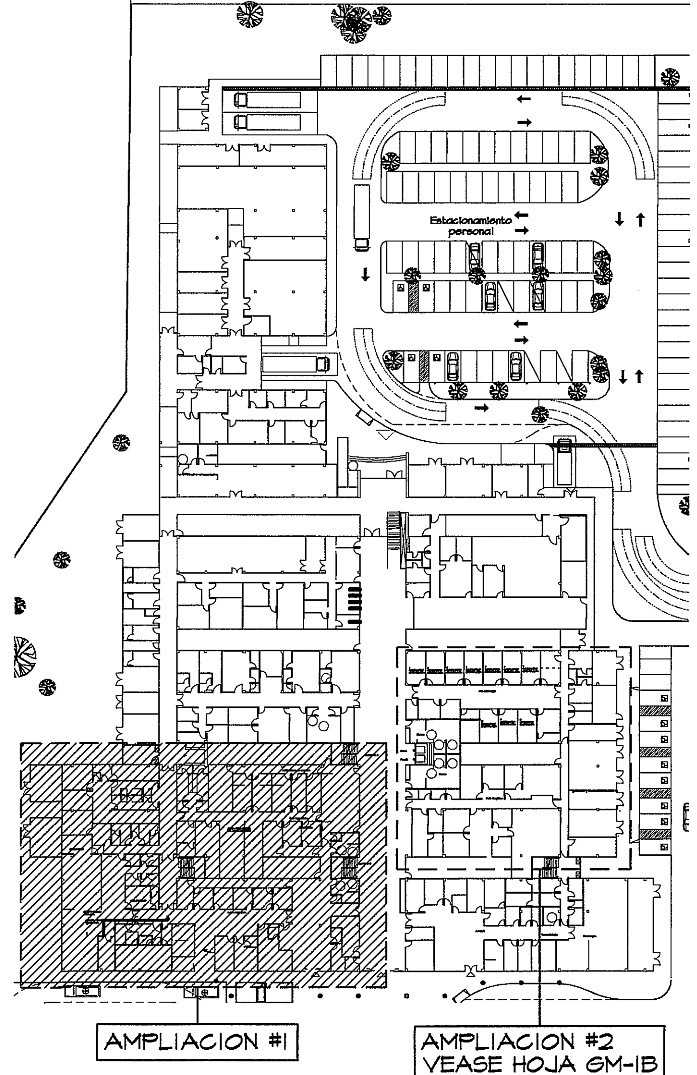
GUIA DE AMPLIACIONES POR ZONAS ESCALA 1:400 PLANTA BAJA
