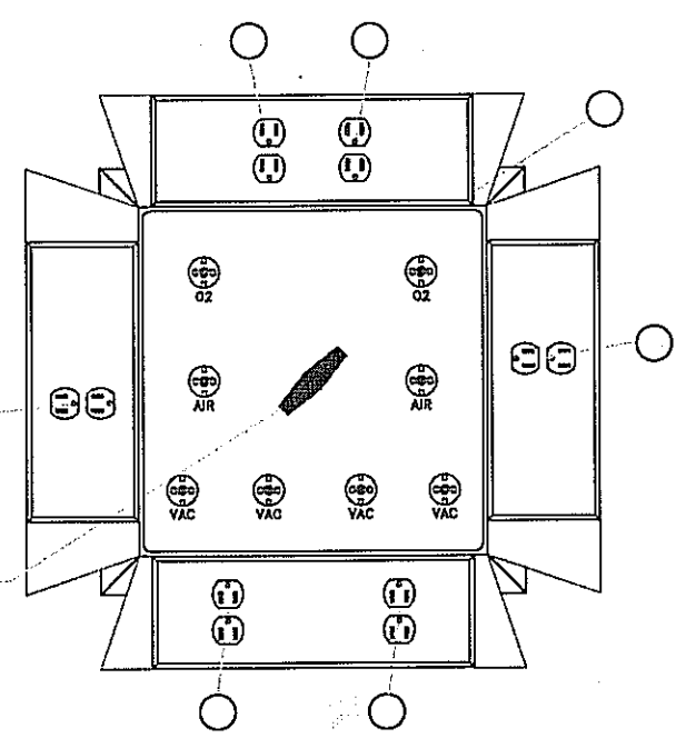
VISTA INFERIOR
