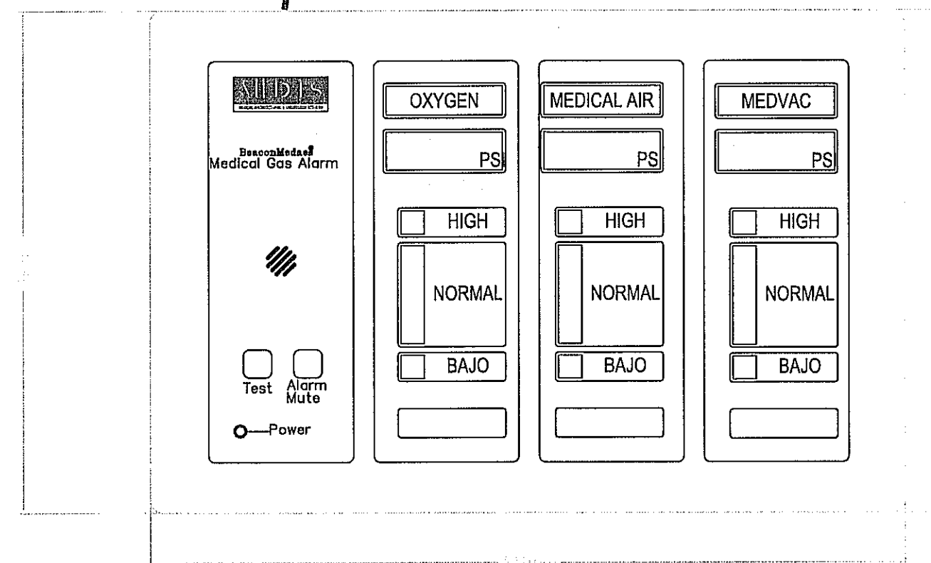
DETALLE FRONTAL
