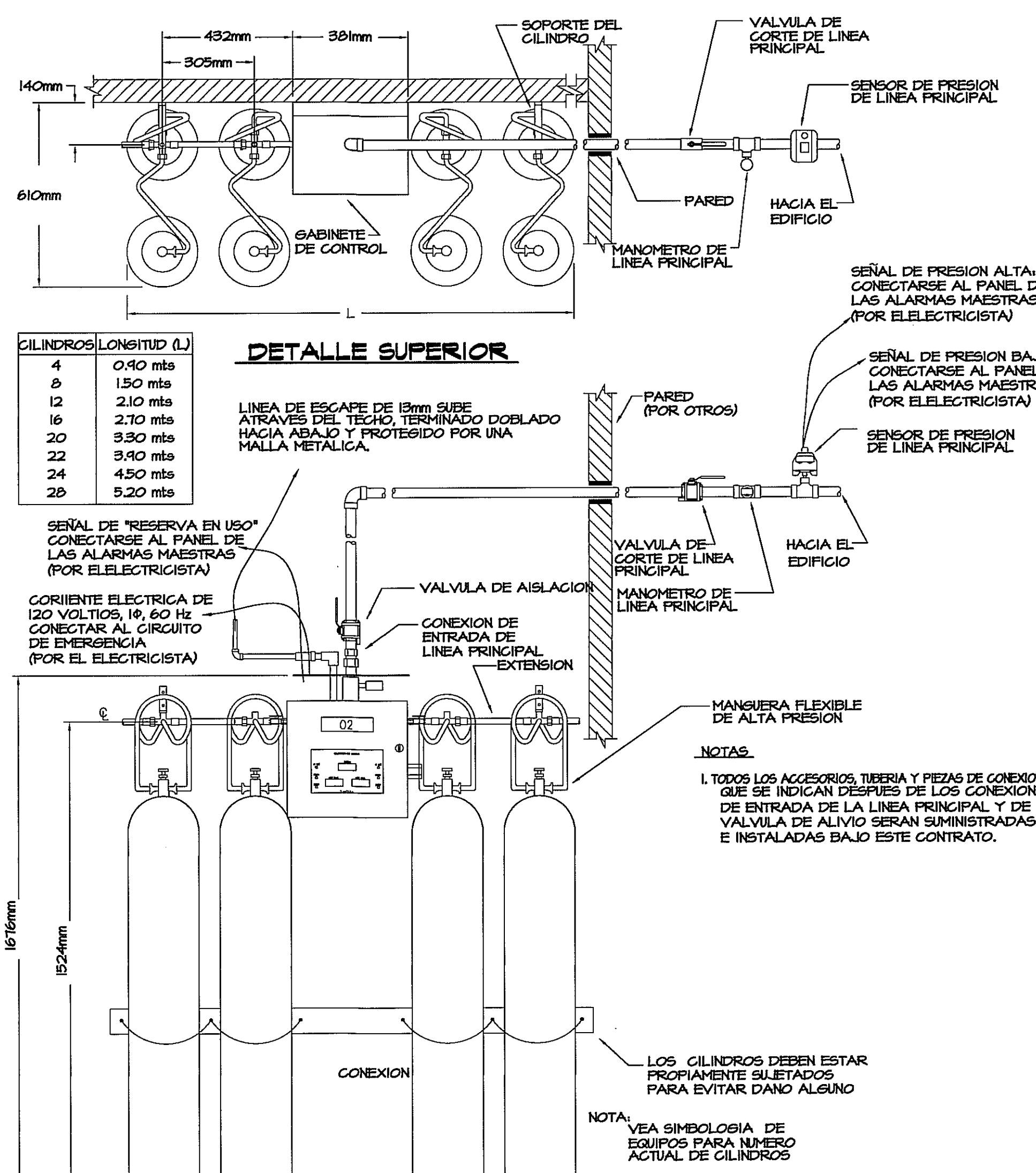
DT-01 MANIFOLD DE GASES MEDICOS (TÍPICO) GM-7 SIN ESCALA
