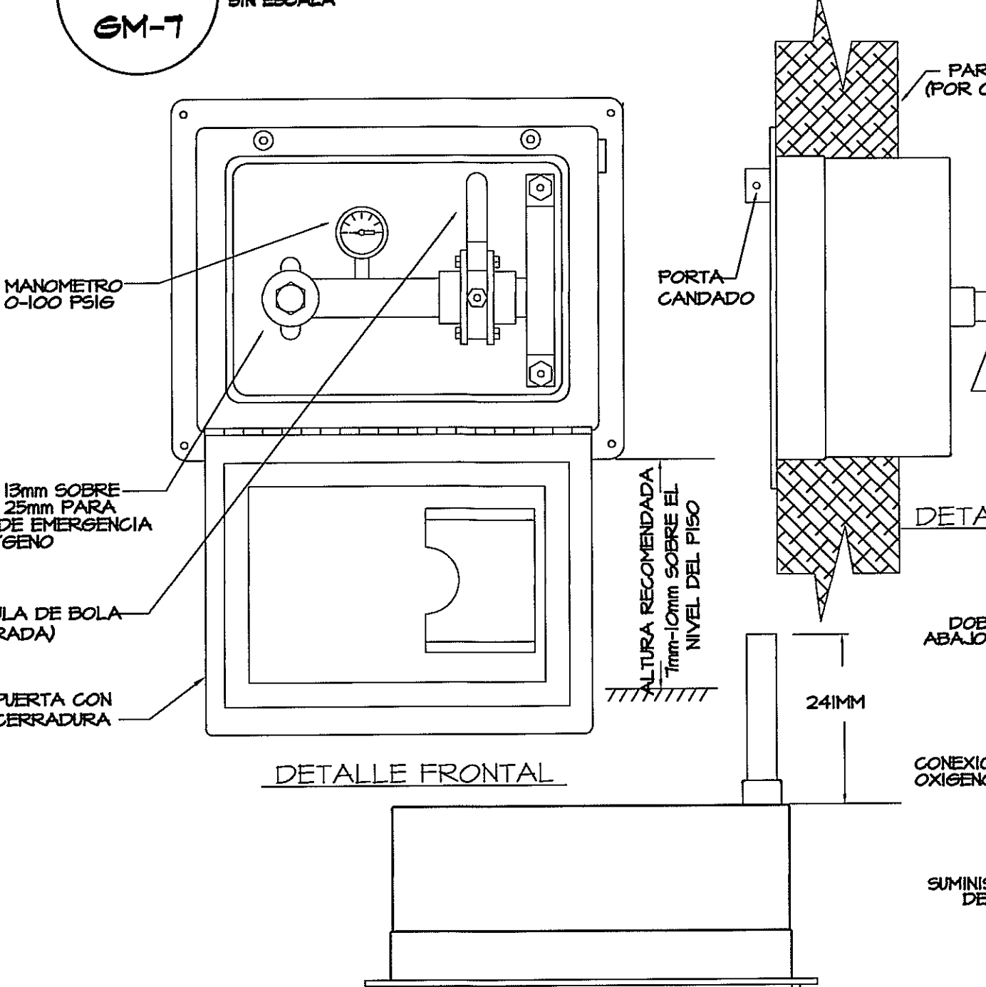
DT-04 ENTRADA DE EMERGENCIA DE OXIGENO "EO" GM-7 SIN ESCALA
