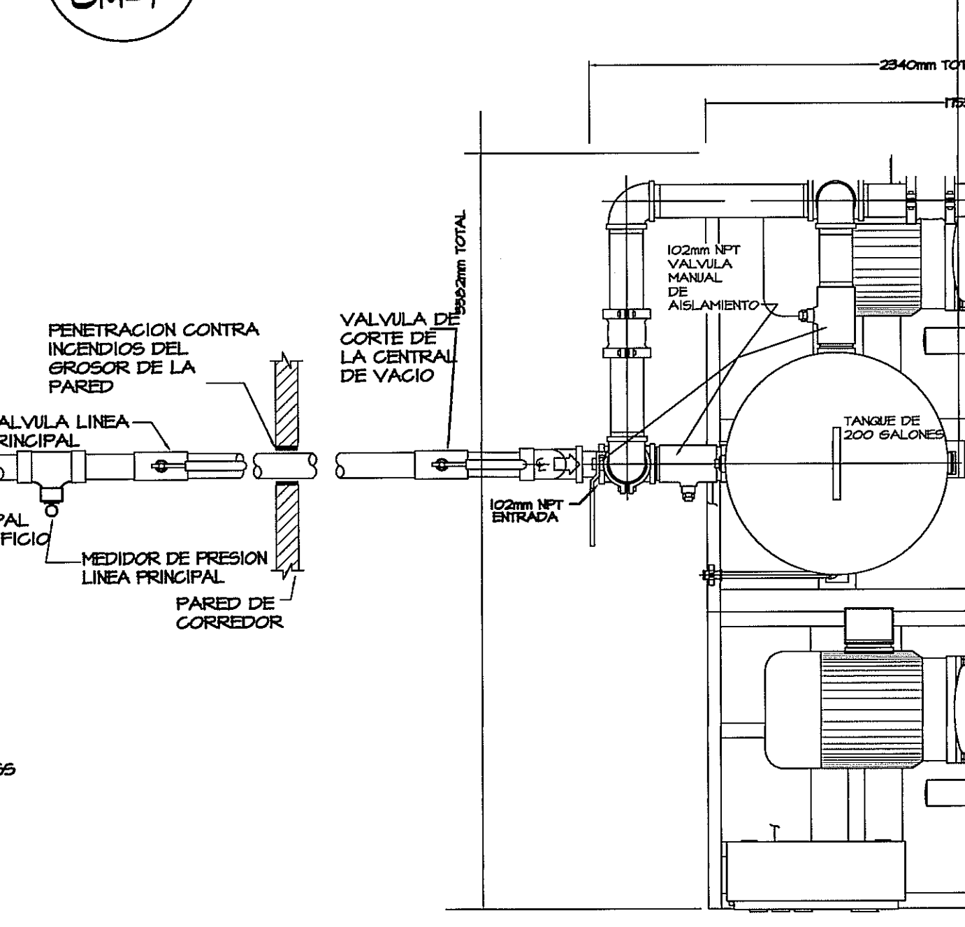
DT-03 BOMBA DE VACIO (3 HP DOBLE) "MVP" (TÍPICO) GM-7 SIN ESCALA
