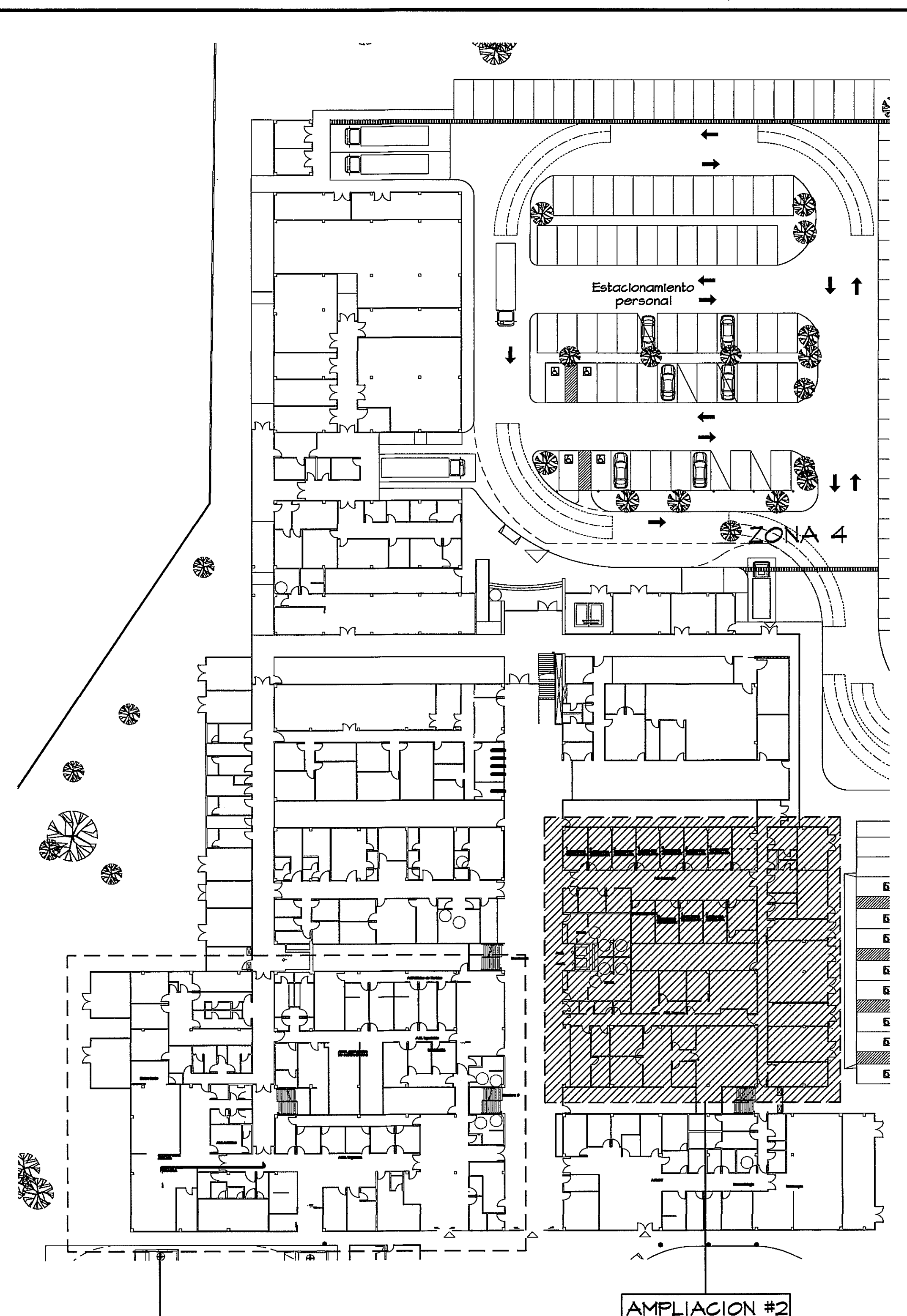
GUÍA DE AMPLIACIONES POR ZONAS ESCALA 1:400 PLANTA BAJA
