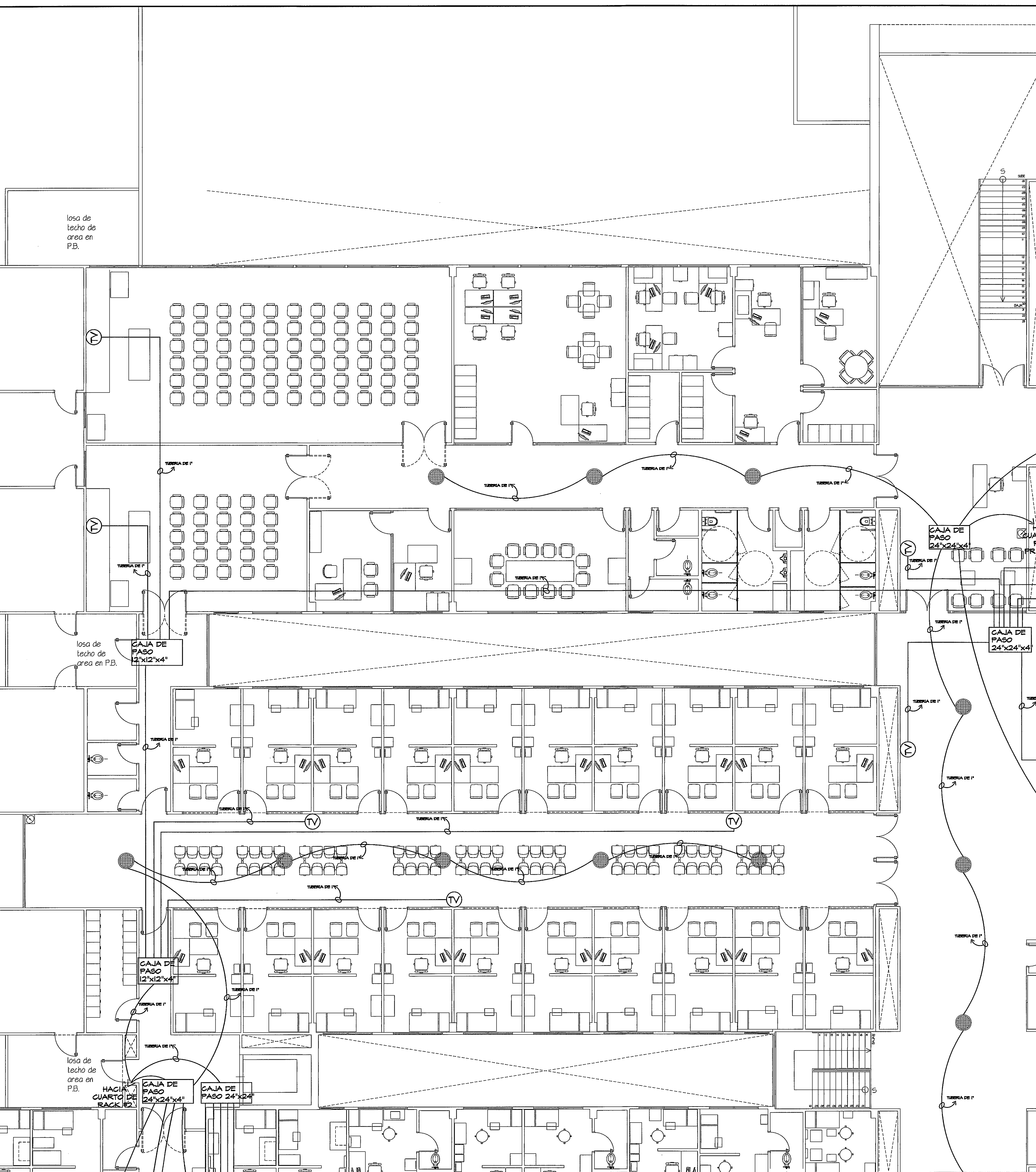
AMPLIACION DE ZONA 6 PLANTA AUDIO - TV (NIVEL 100) ESCALA.- 1/75
