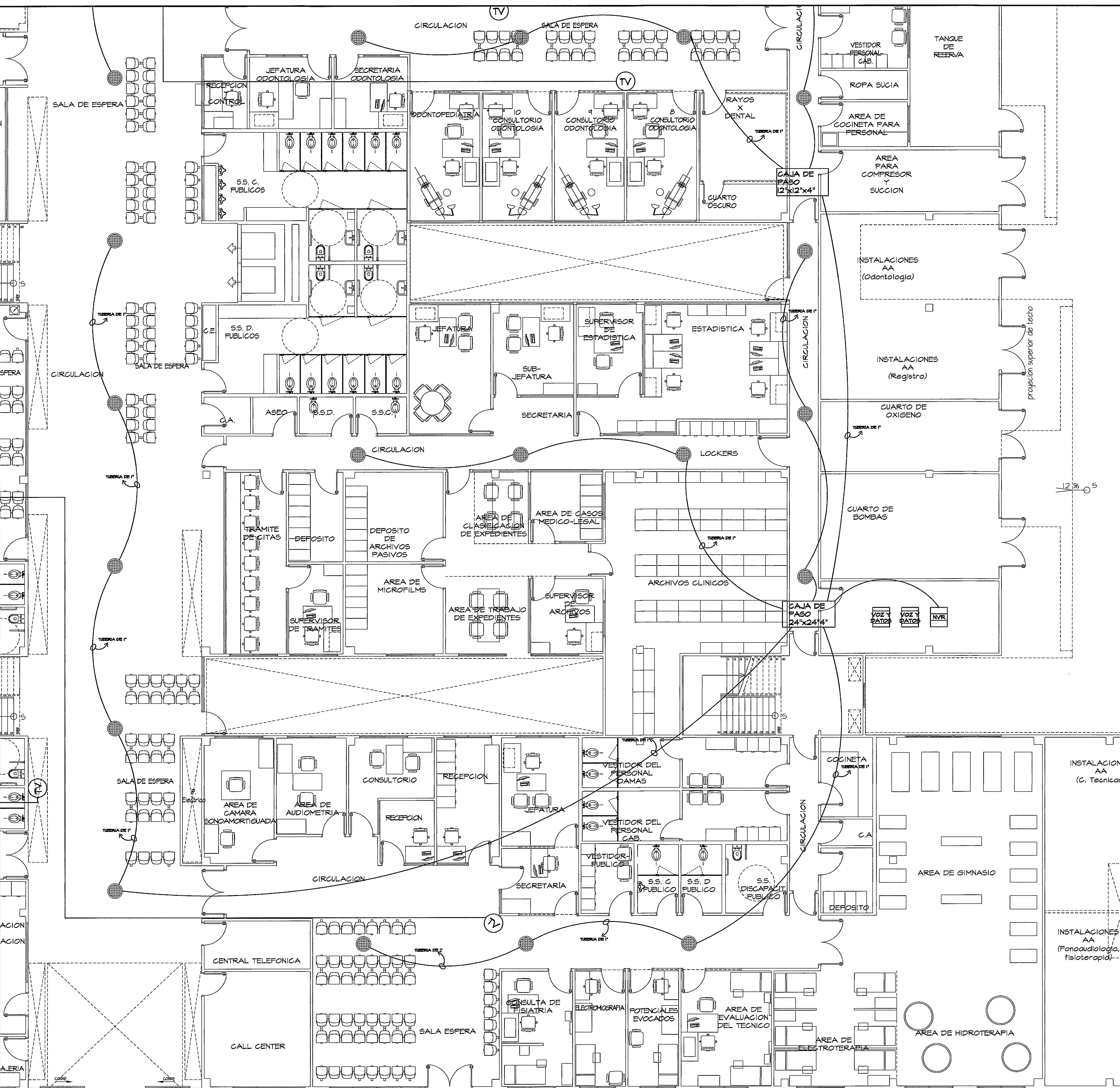
VER AMPLIACION DE ZONA 1 HOJA SE-03A VER AMPLIACION DE ZONA 4 HOJA SE-03D VER AMPLIACION DE ZONA 2 HOJA SE-03B VER AMPLIACION DE ZONA 3 HOJA SE-03C GUÍA DE AMPLIACIONES POR ZONAS ESCALA.- 1/400 PLANTA DE AUDIO - TV
