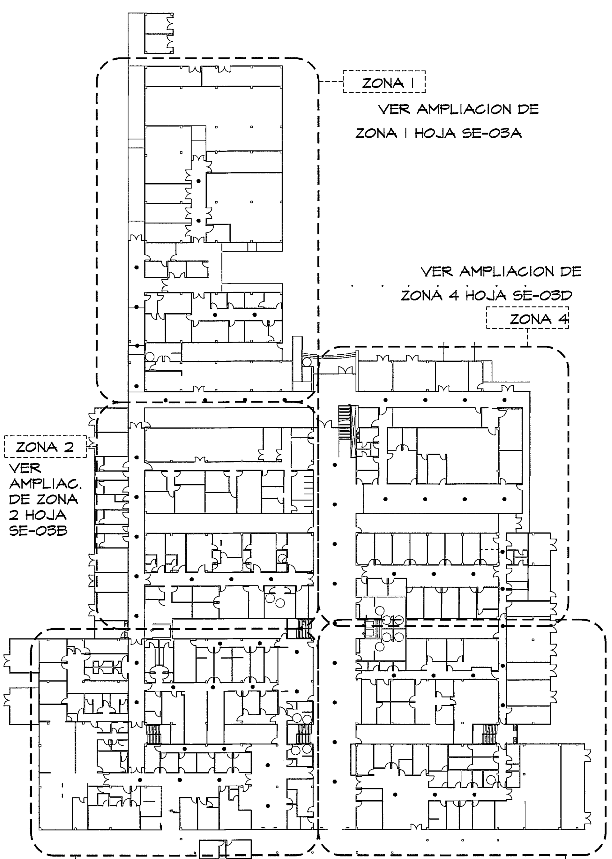
VER AMPLIACION DE ZONA 1 HOJA SE-03A VER AMPLIACION DE ZONA 4 HOJA SE-03D VER AMPLIACION DE ZONA 2 HOJA SE-03B VER AMPLIACION DE ZONA 3 HOJA SE-03C GUÍA DE AMPLIACIONES POR ZONAS ESCALA.- 1/400 PLANTA DE AUDIO - TV
