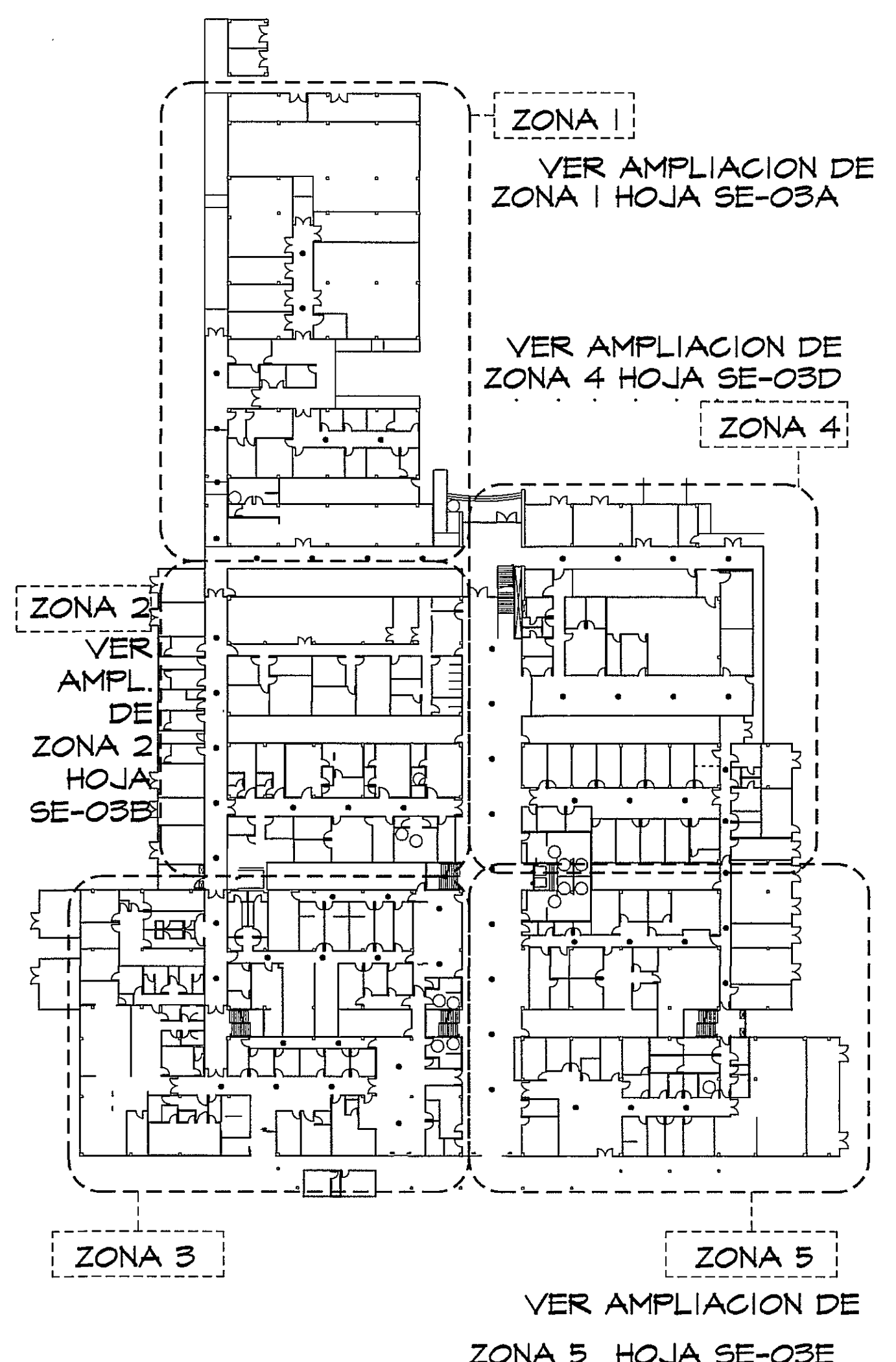
GUÍA DE AMPLIACIONES POR ZONAS ESCALA.- 1/600 PLANTA DE AUDIO - TV
