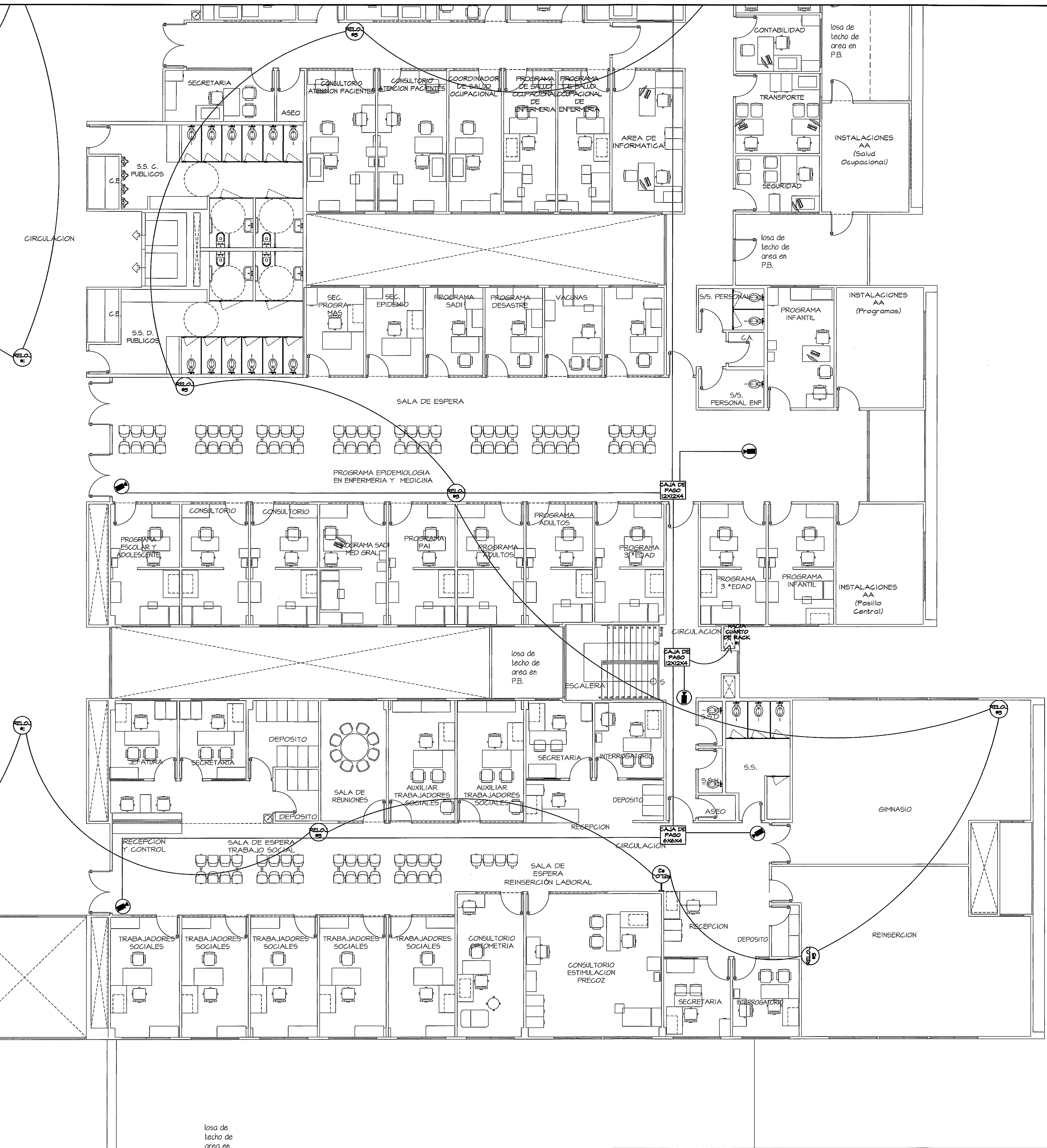
AMPLIACION DE ZONA 9 PLANTA ALTA ESCALA.- 1/75
