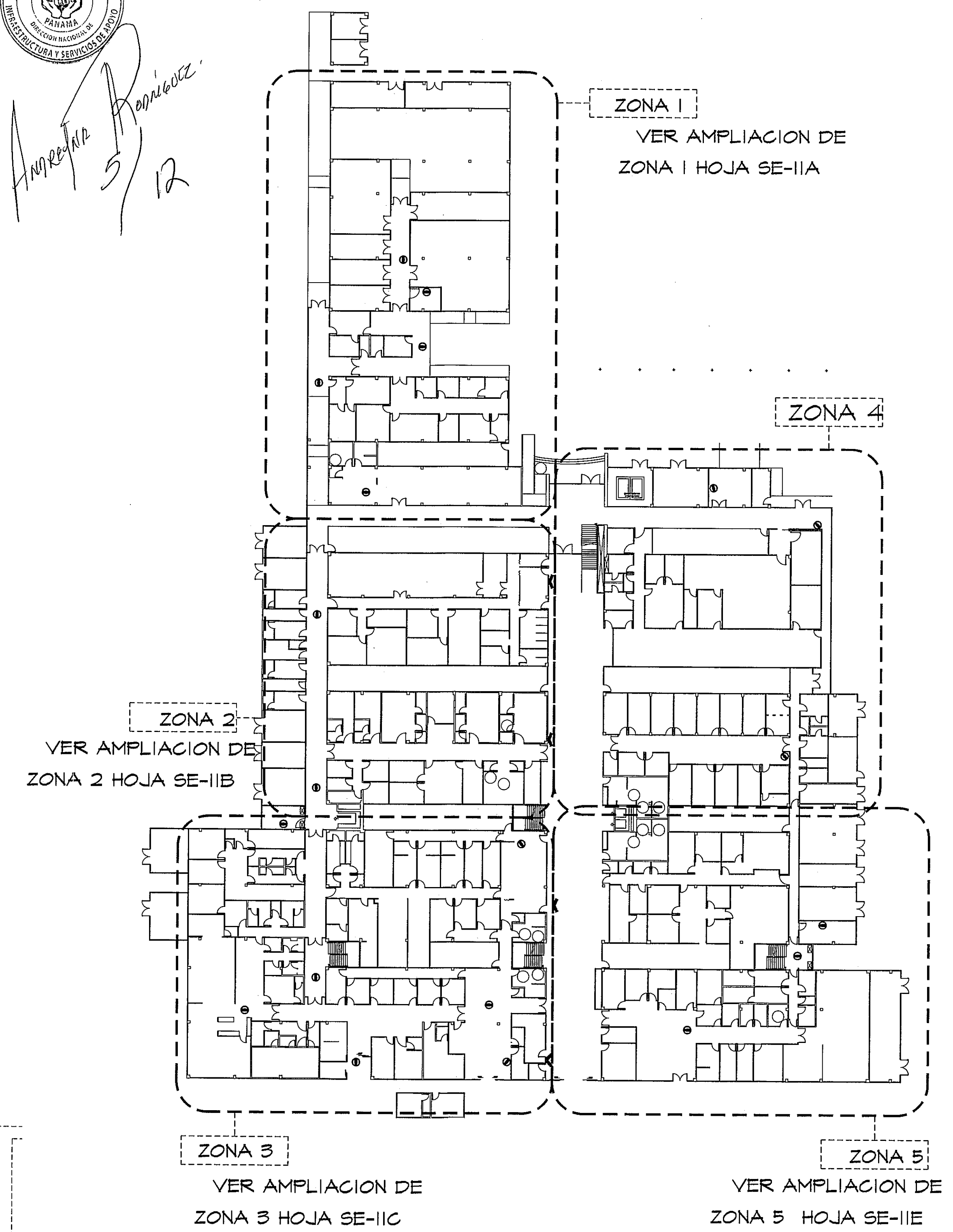
GUIA DE AMPLIACIONES POR ZONAS ESCALA.- 1/400 PLANTA RELOJ -CCTV
