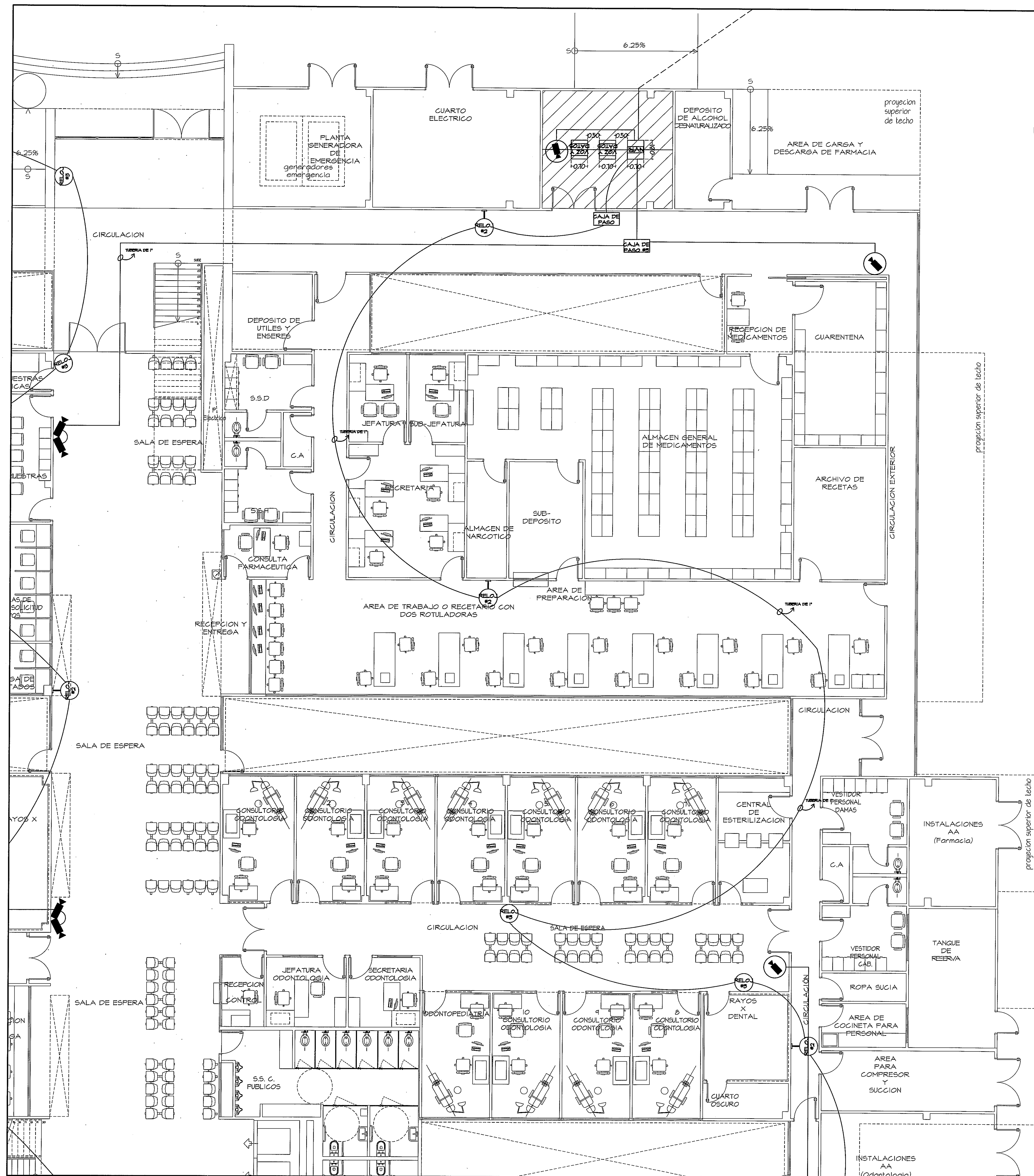
AMPLIACION DE ZONA 4 PLANTA RELOJ - CCTV (NIVEL 000) ESCALA.- 1/75
