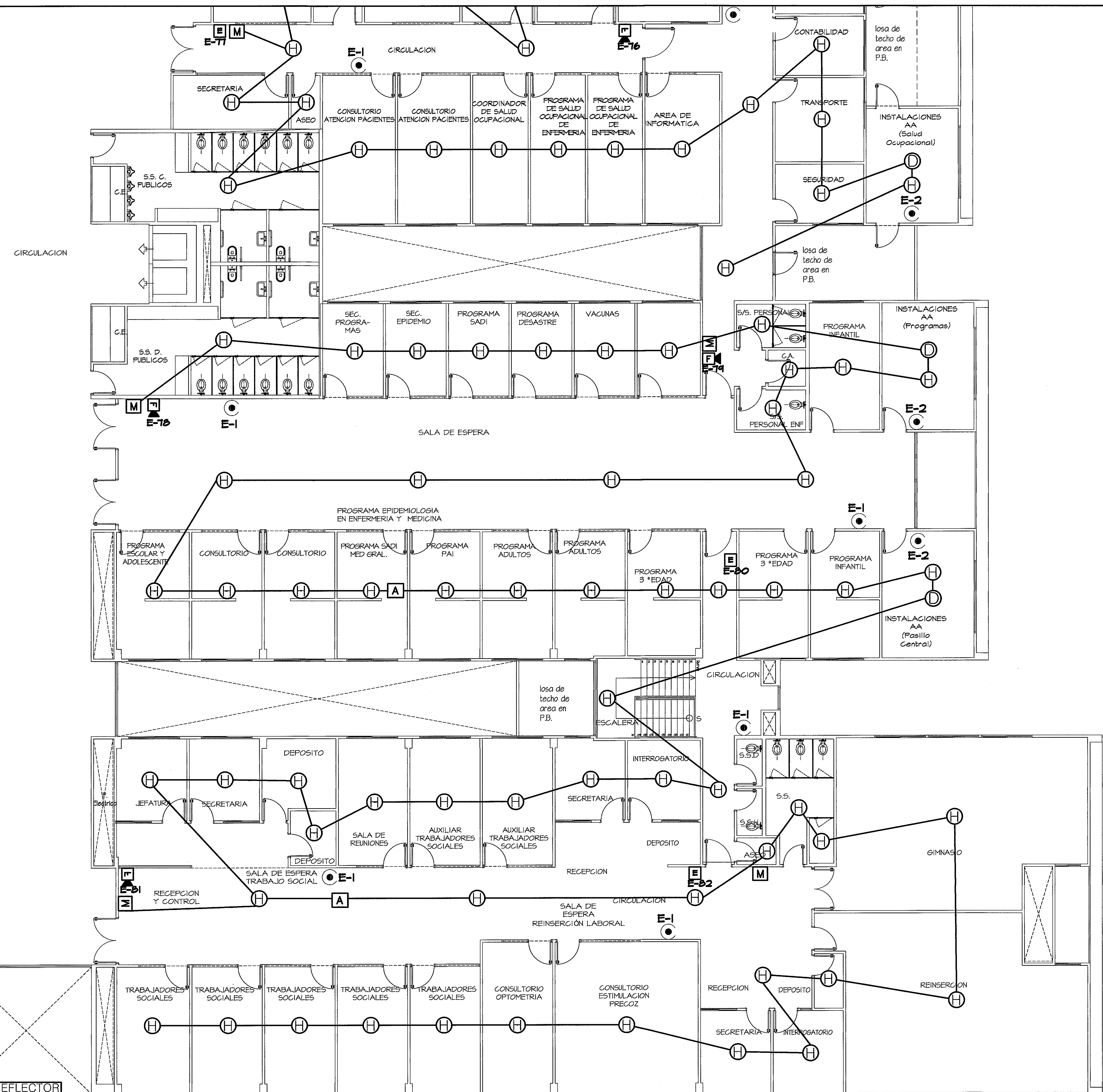
VER AMPLIACION DE ZONA 6 HOJA SE-02A VER AMPLIACION DE ZONA 8 HOJA SE-02C VER AMPLIACION DE ZONA 7 HOJA SE-02B GUÍA DE AMPLIACIONES POR ZONAS ESCALA.- 1/400 PLANTA ALTA INCENDIO
