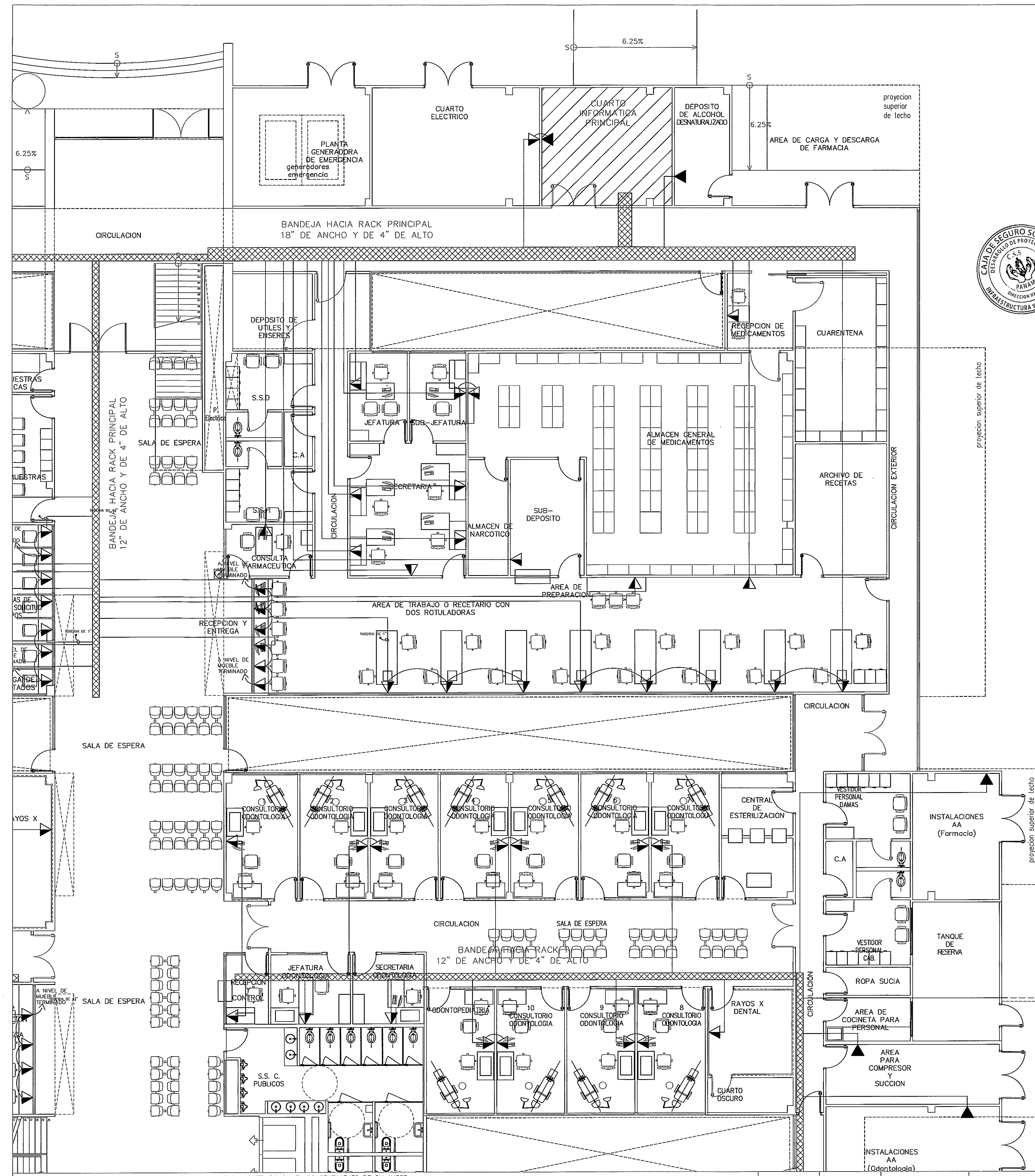
AMPLIACION DE ZONA 4 PLANTA VOZ Y DATOS (NIVEL 000) ESCALA.- 1/75
