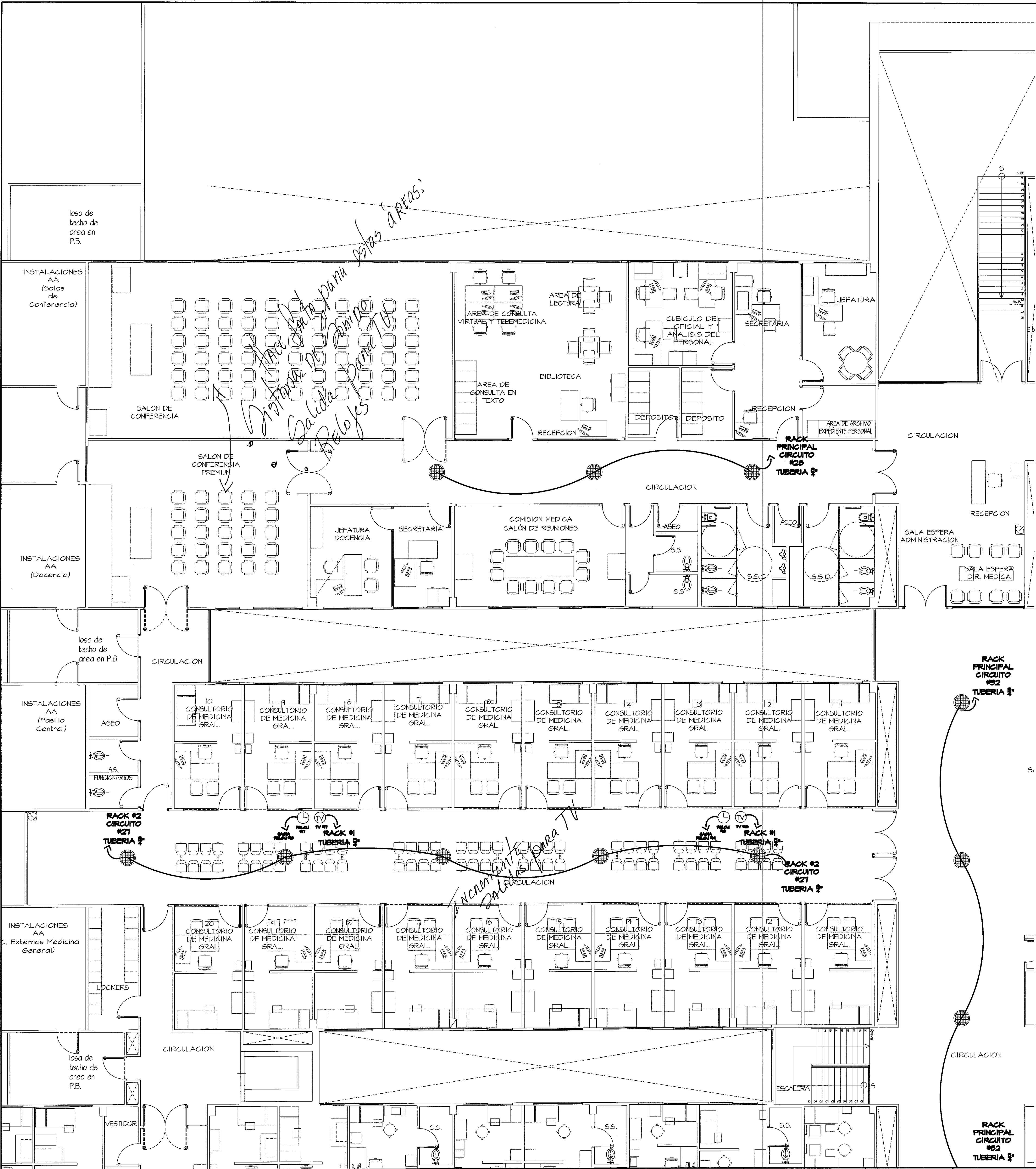
AMPLIACION DE ZONA 6 PLANTA AUDIO- RELOJ- TV (NIVEL 100) ESCALA.- 1/75
