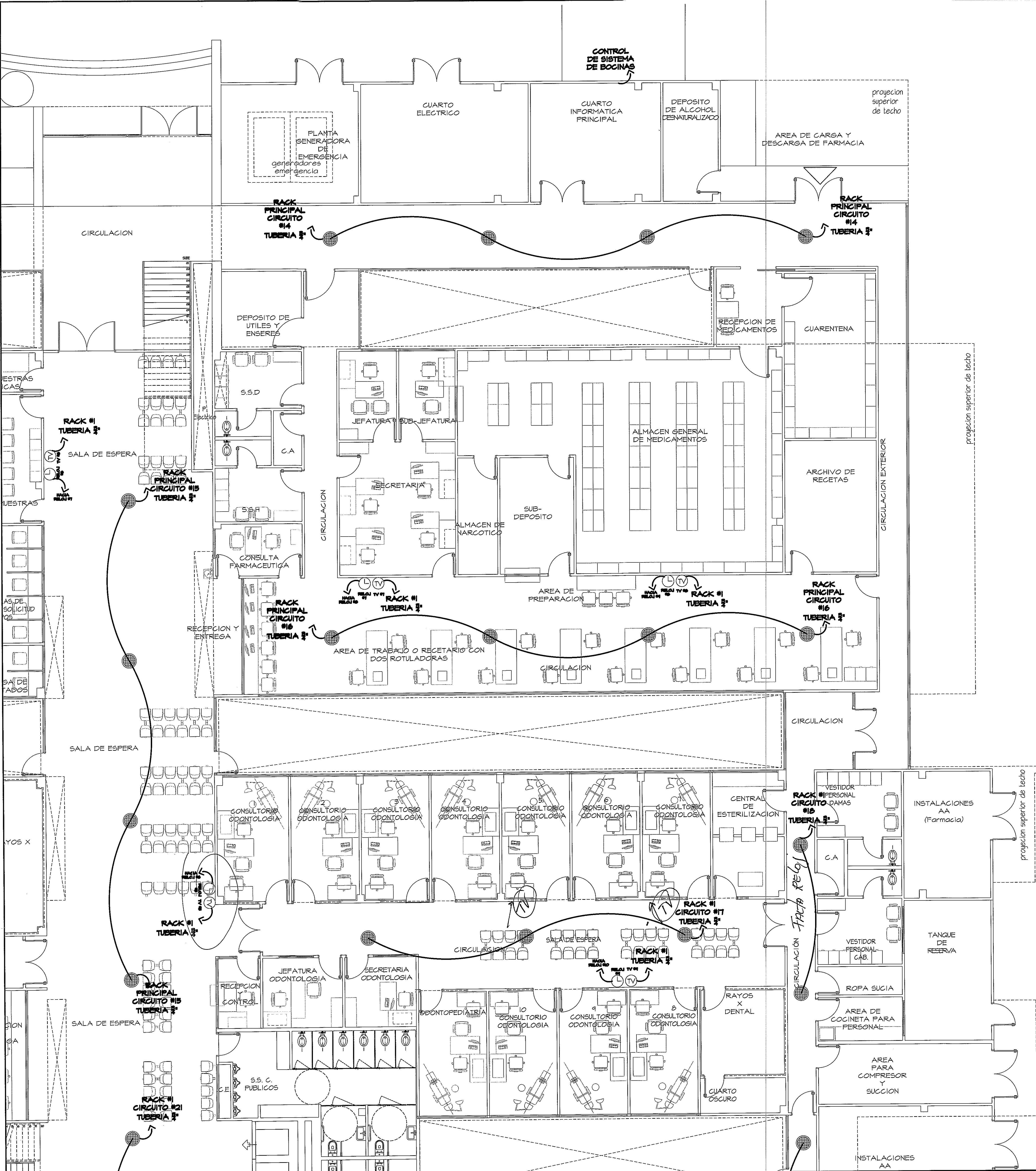
AMPLIACION DE ZONA 4 PLANTA AUDIO- RELOJ- TV (NIVEL 000) ESCALA: - 1/75
