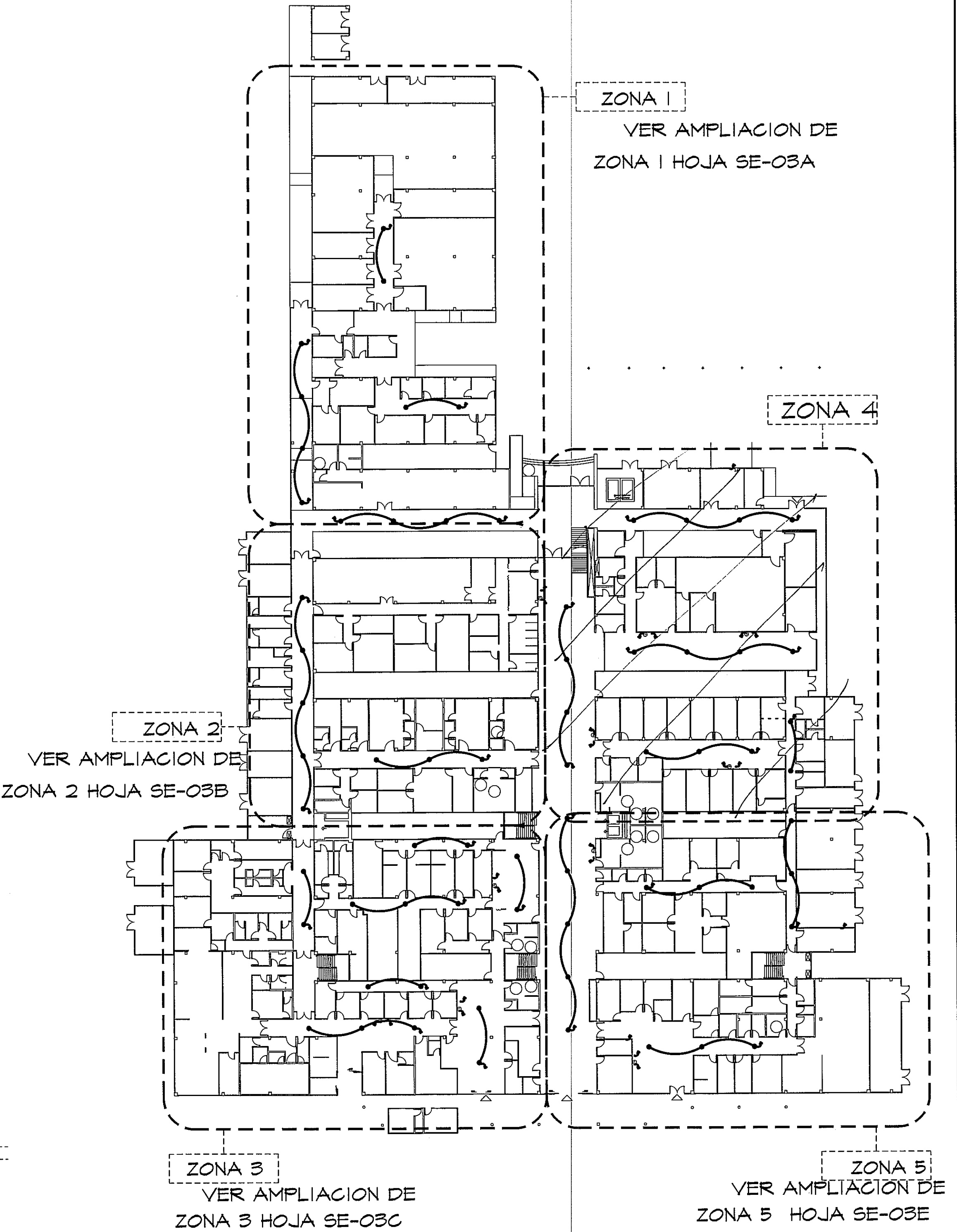
GUÍA DE AMPLIACIONES POR ZONAS ESCALA: - 1/400 PLANTA DE AUDIO-RELOJ-TV
