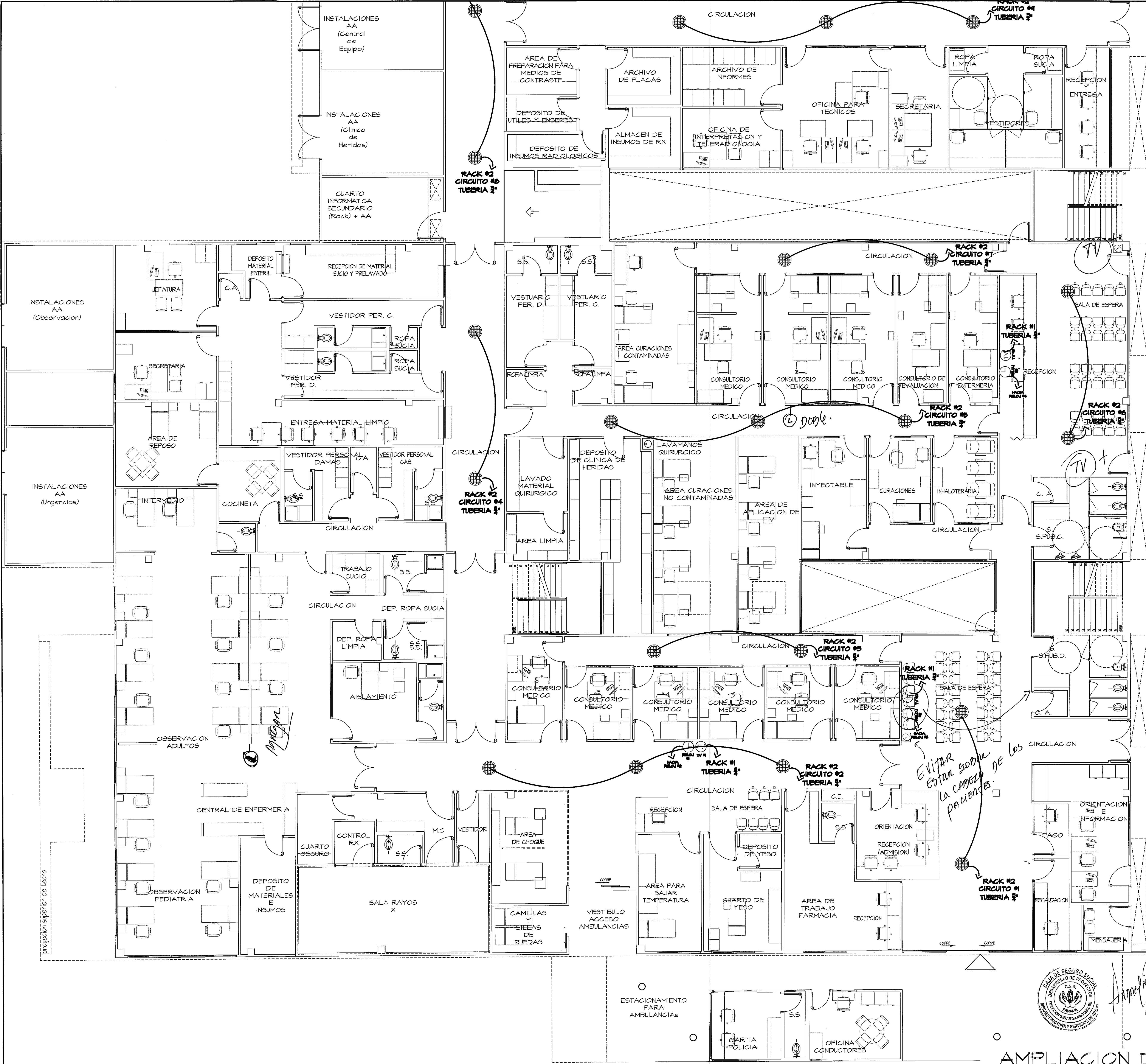
GUIA DE AMPLIACIONES POR ZONAS ESCALA.- 1/600 PLANTA DE AUDIO-RELOJ-TV
