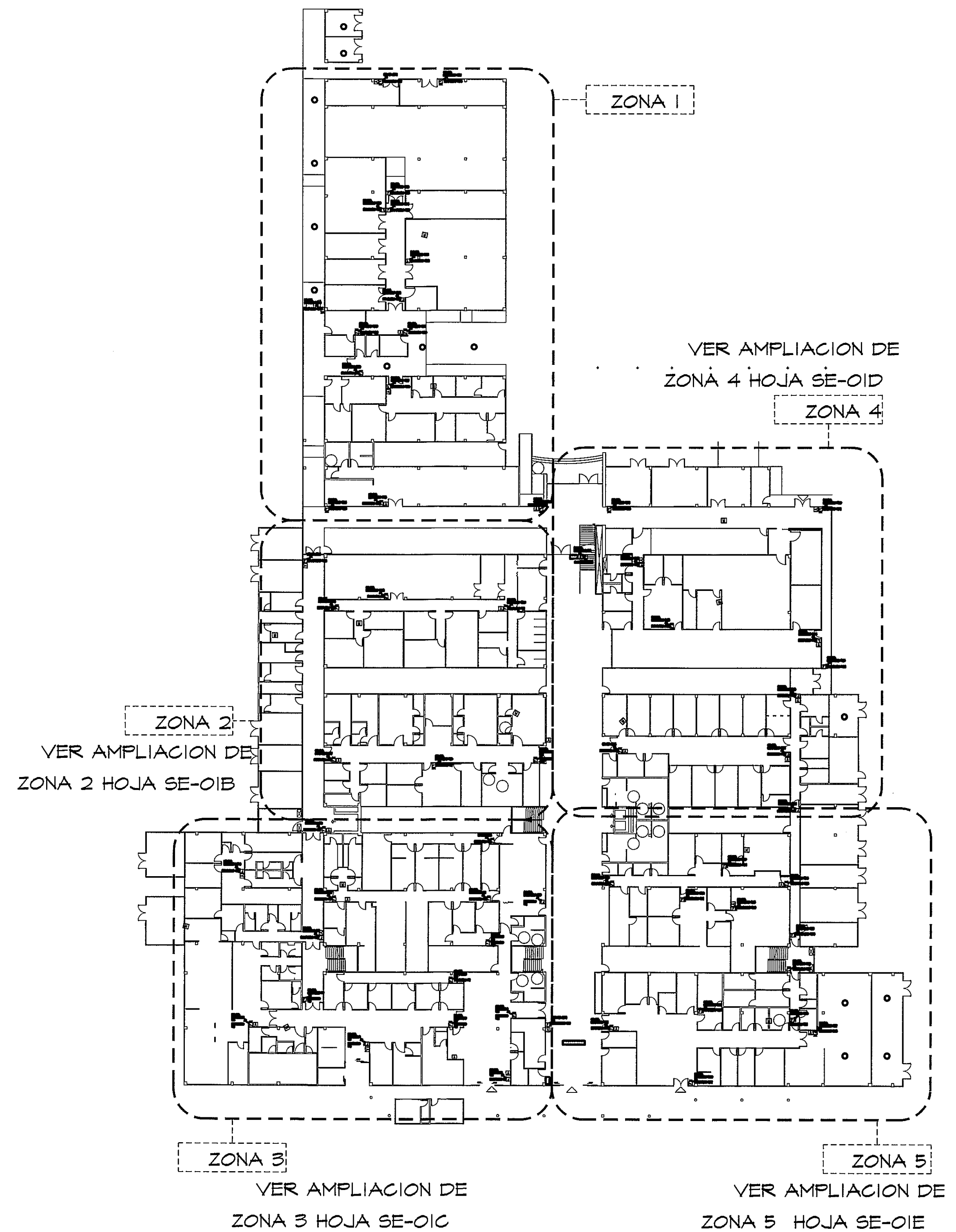
GUIA DE AMPLIACIONES POR ZONAS ESCALA.- 1/400 PLANTA DE INCENDIO
