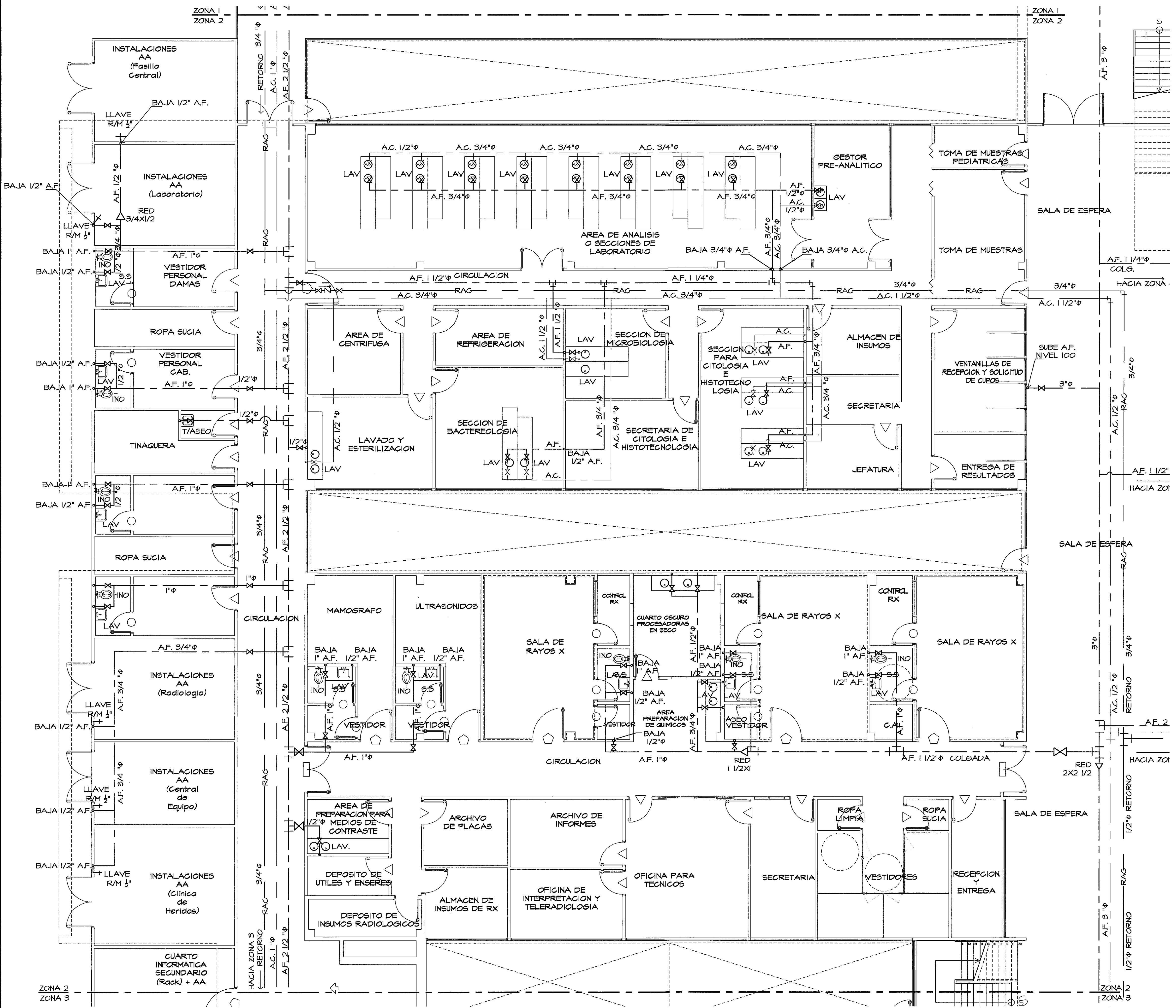
PLANTA AMPLIACION ZONA 2 SISTEMA AGUA POTABLE - NIVEL 000 ESCALA 1:75
