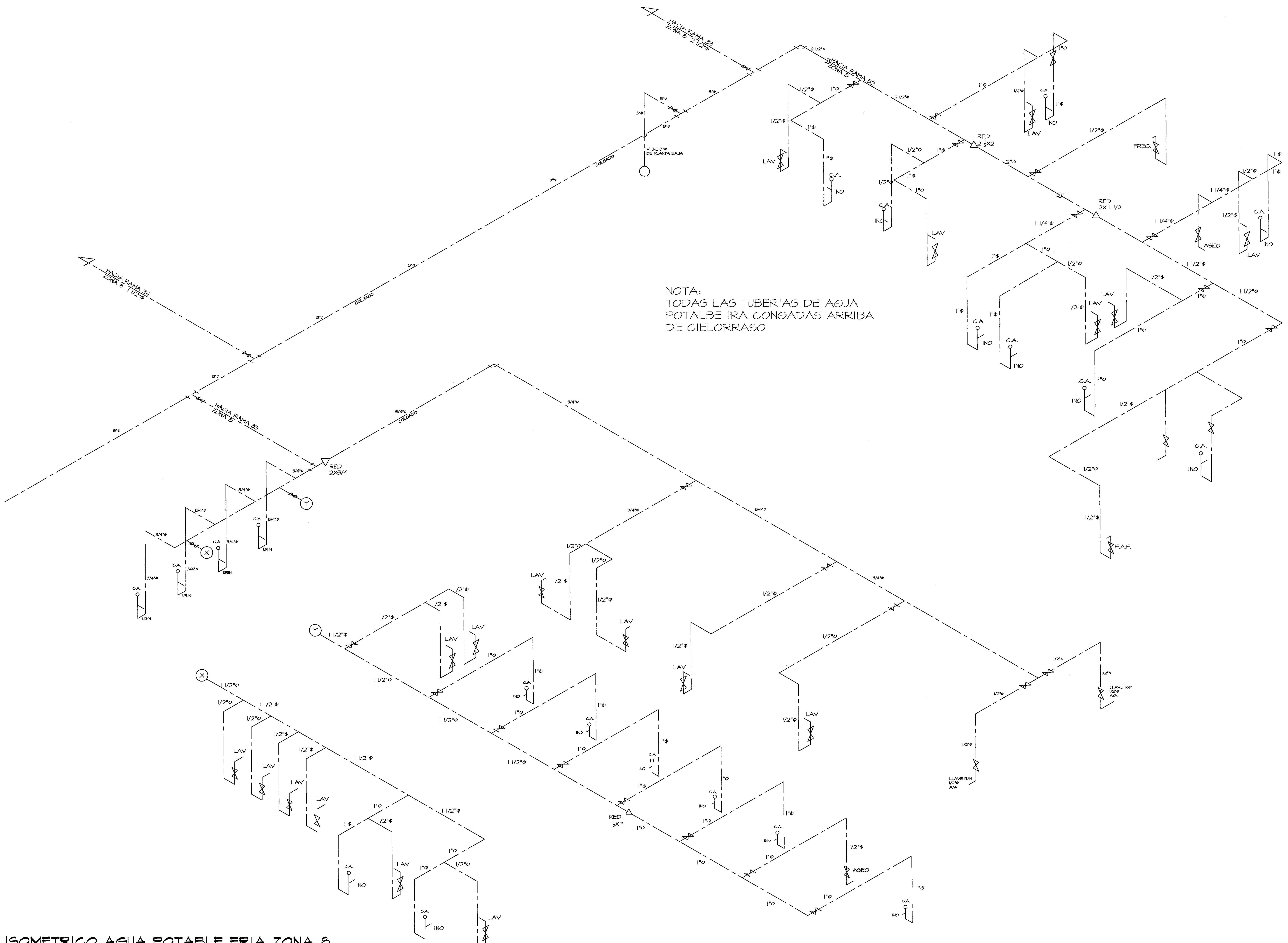
ISOMETRICO AGUA POTABLE FRIA ZONA 8 SIN ESCALA
