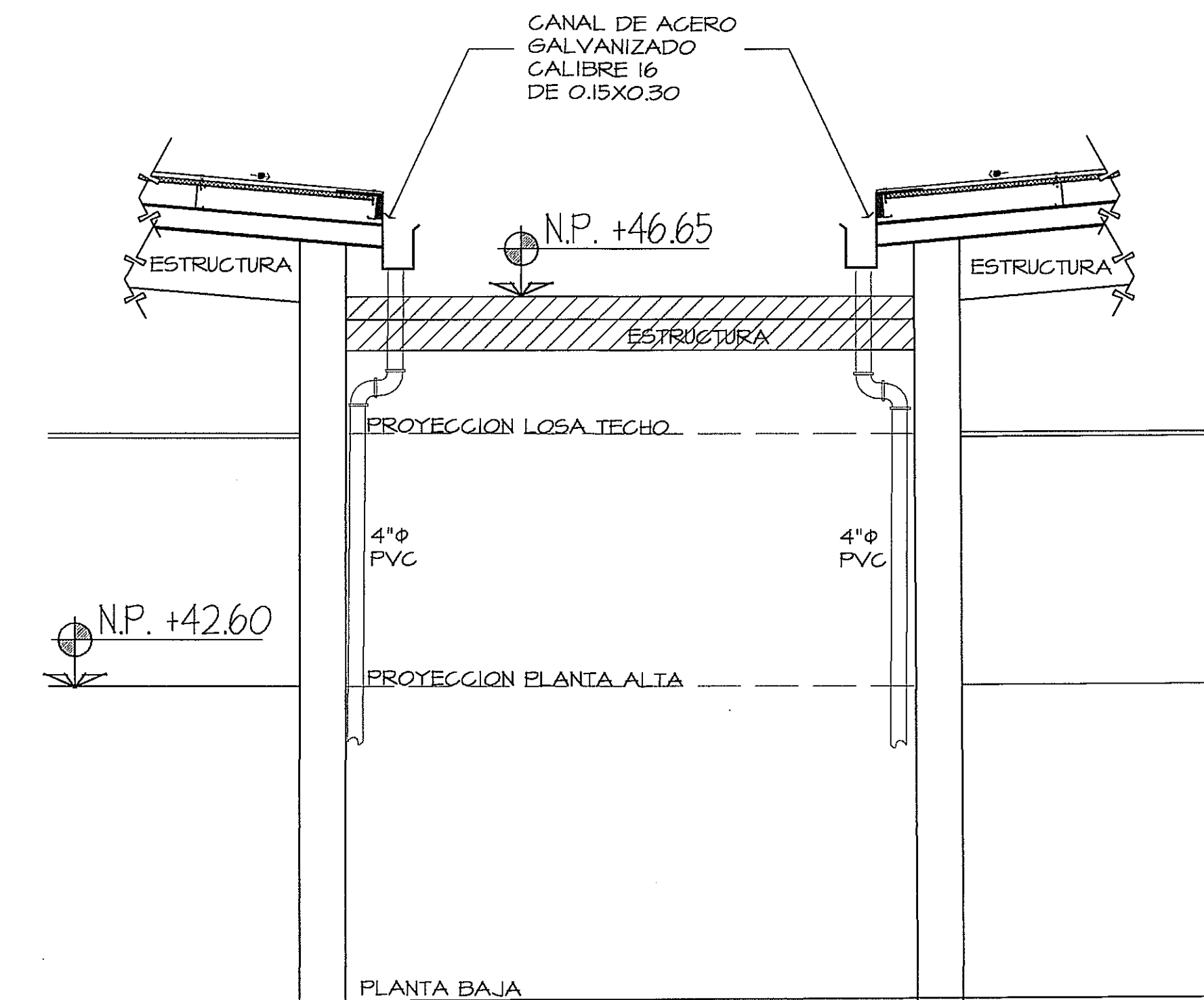
DETALLE SIN ESCALA
