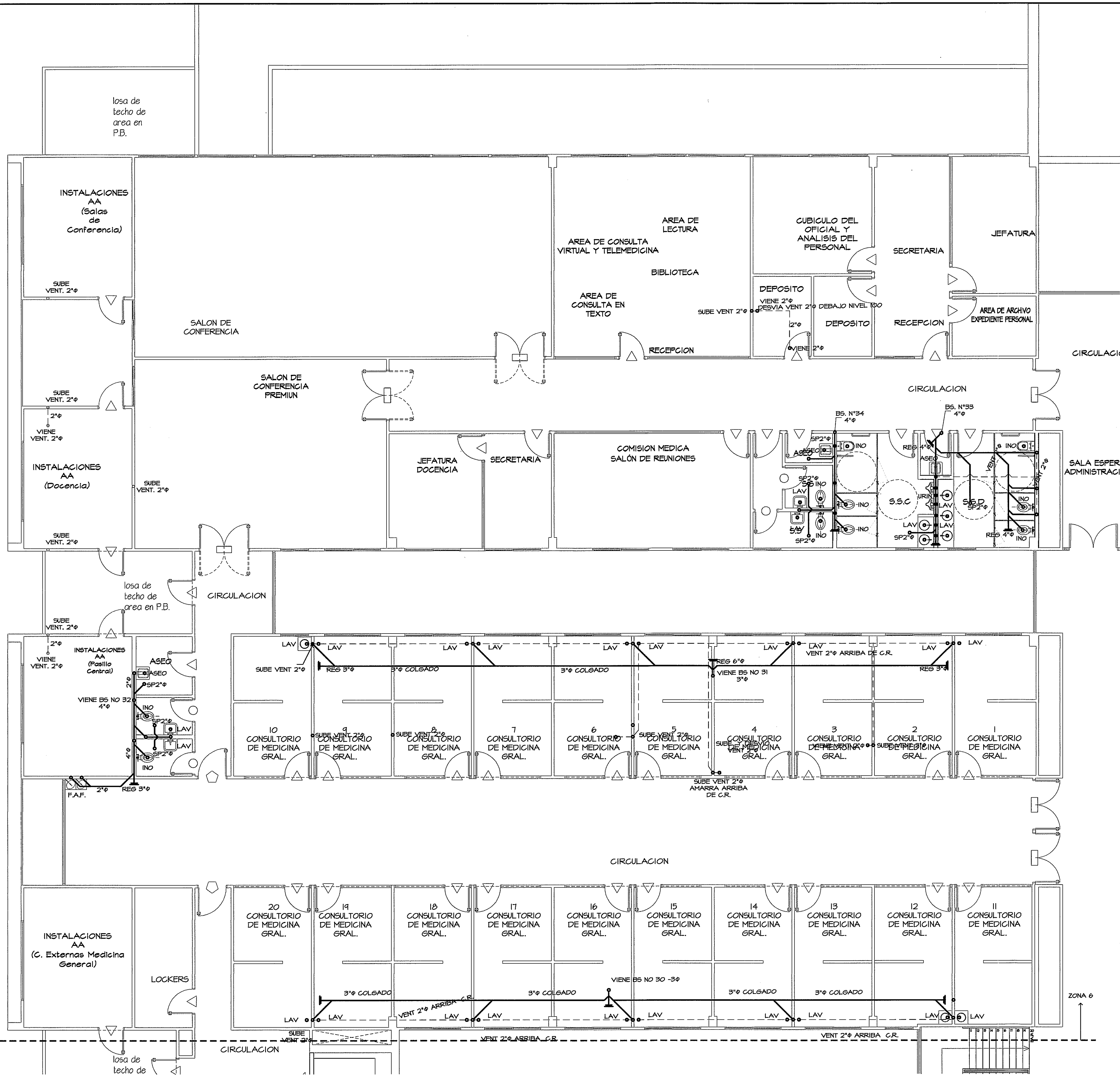
PLANTA AMPLIACION ZONA 6 SANITARIA Y PLUVIAL ESCALA 1:75 PLANTA NIVEL 100
