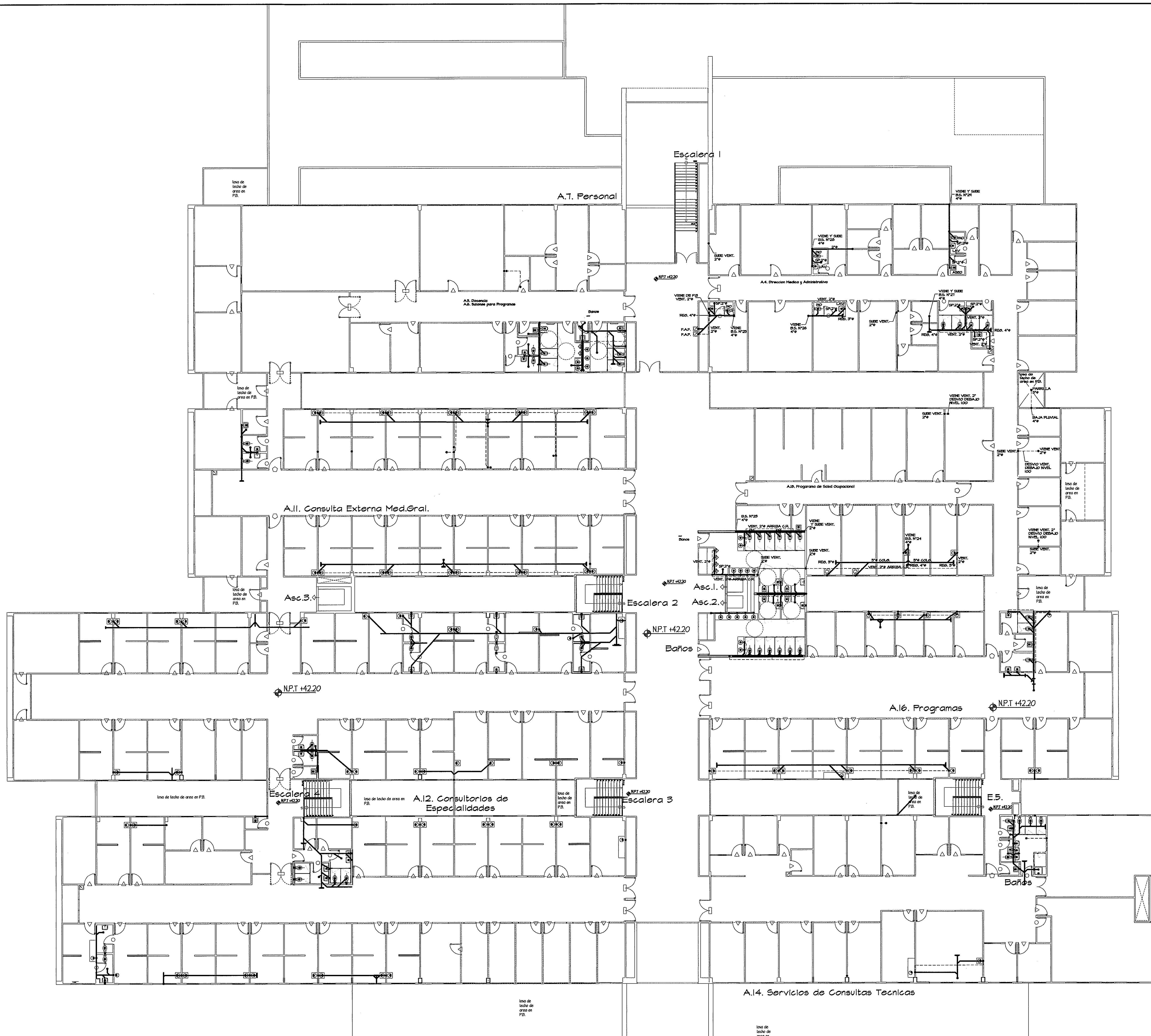
PLANTA GENERAL DE SISTEMA SANITARIO NIVEL 100 ESCALA 1:150
