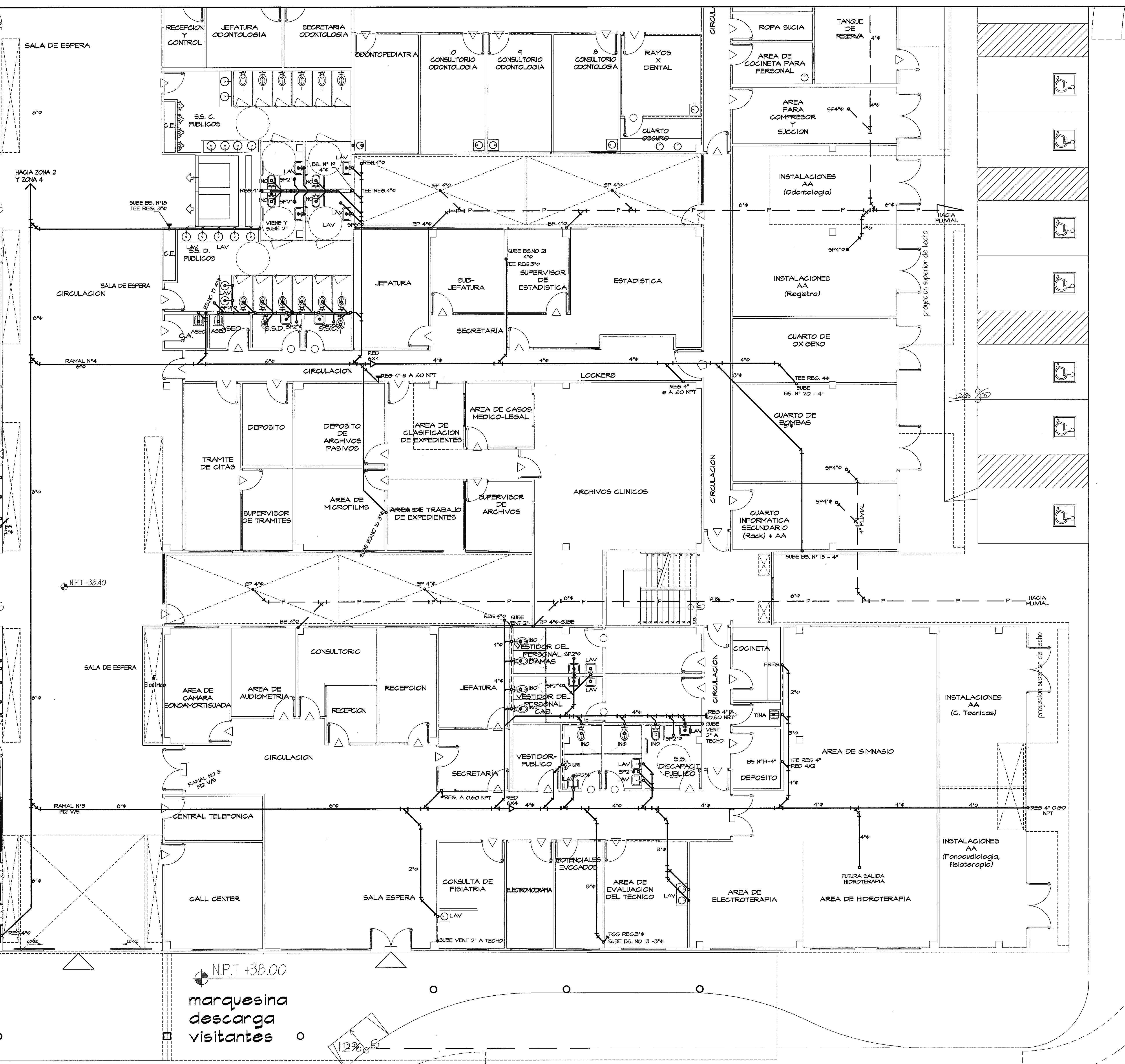
PLANTA AMPLIACION ZONA 5 SANITARIA ESCALA 1:75 PLANTA BAJA
