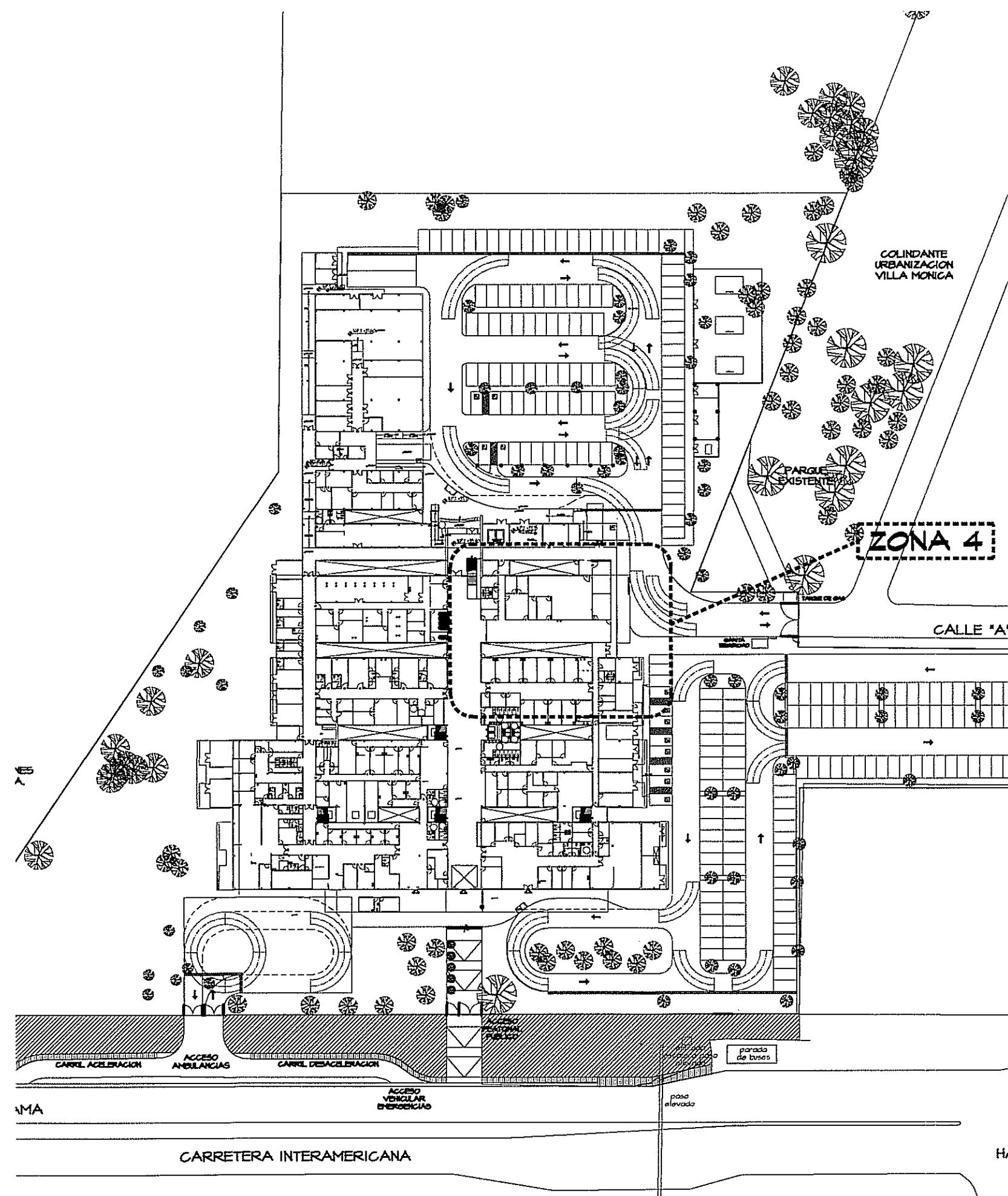
GUIA DE AMPLIACIONES DE ZONAS ESCALA 1:1000 PLANTA BAJA
