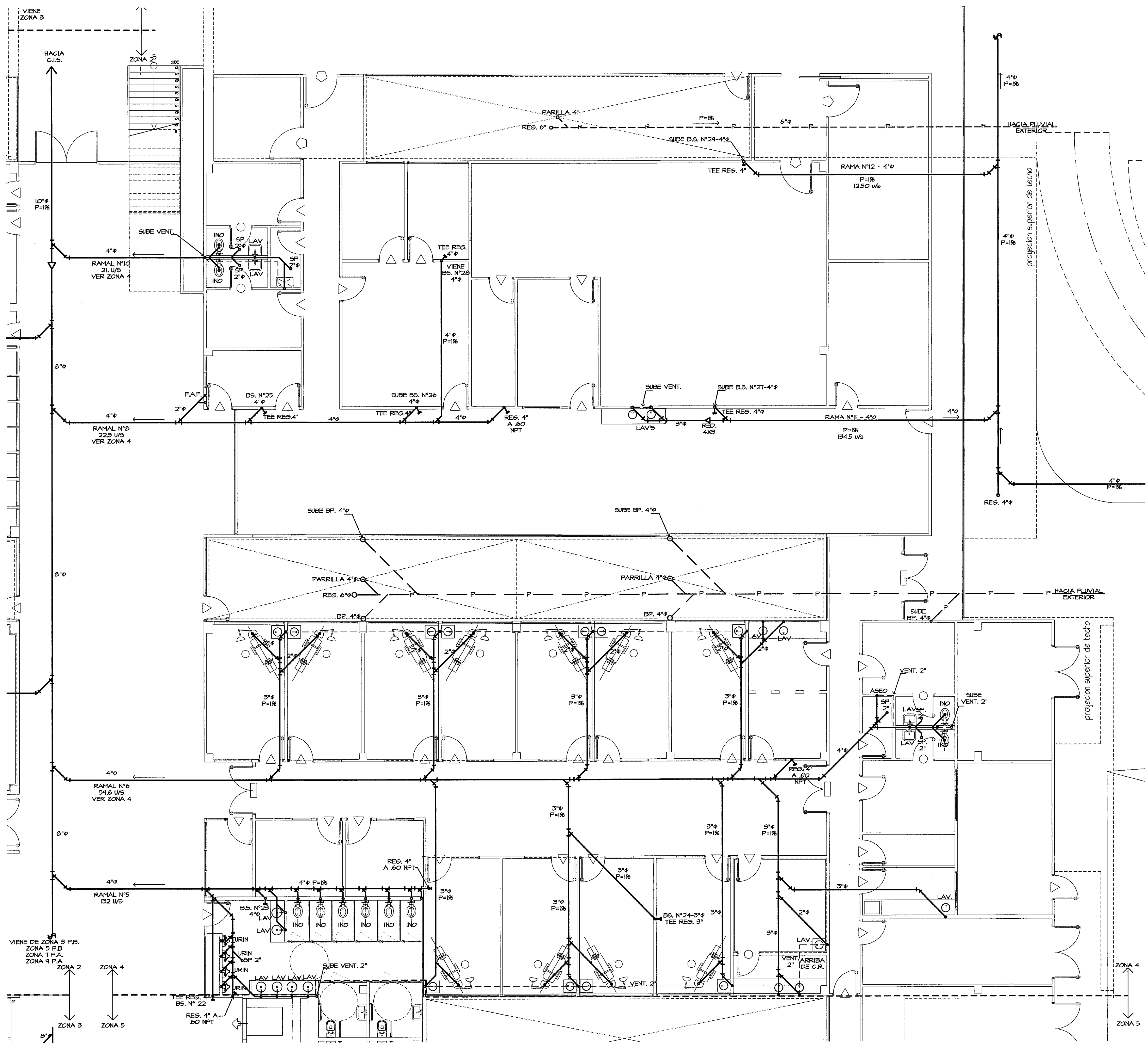
PLANTA AMPLIACION ZONA 4 SANITARIA Y PLUVIAL ESCALA 1:175 PLANTA BAJA
