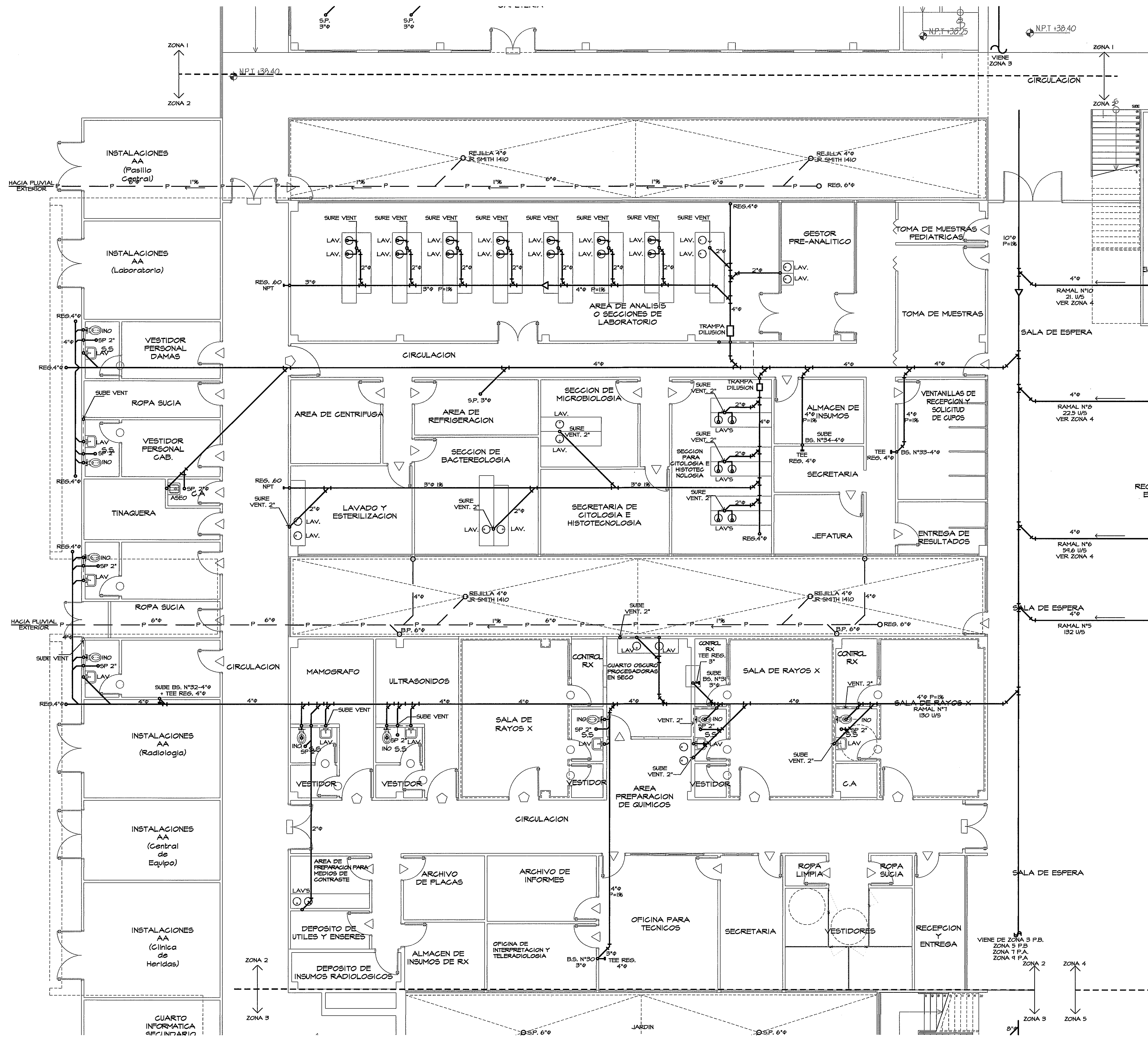
PLANTA AMPLIACION ZONA 2 SANITARIA Y PLUVIAL ESCALA 1:75 PLANTA BAJA
