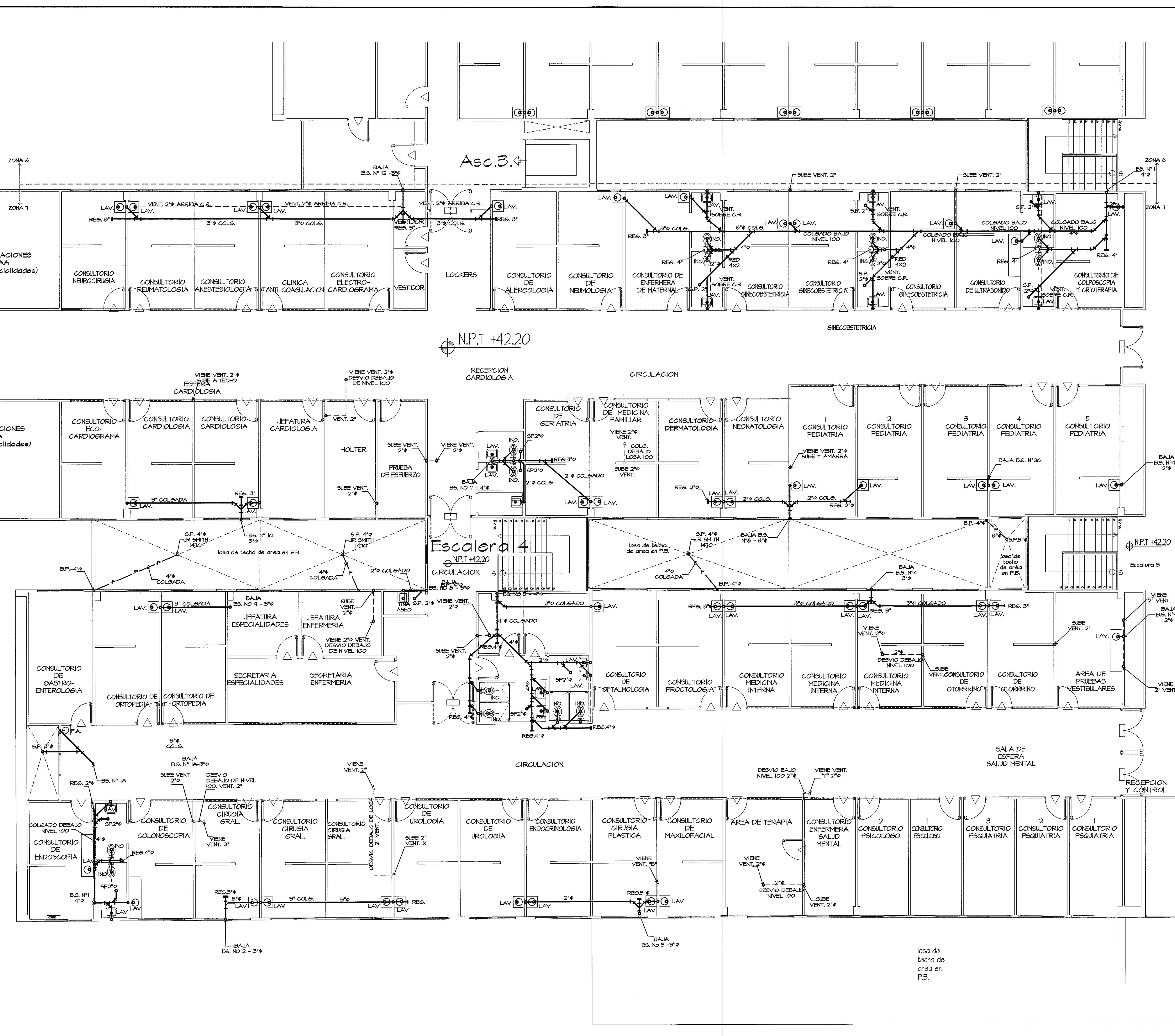
PLANTA AMPLIACION ZONA 7 SANITARIA ESCALA 1:75 PLANTA NIVEL 100
