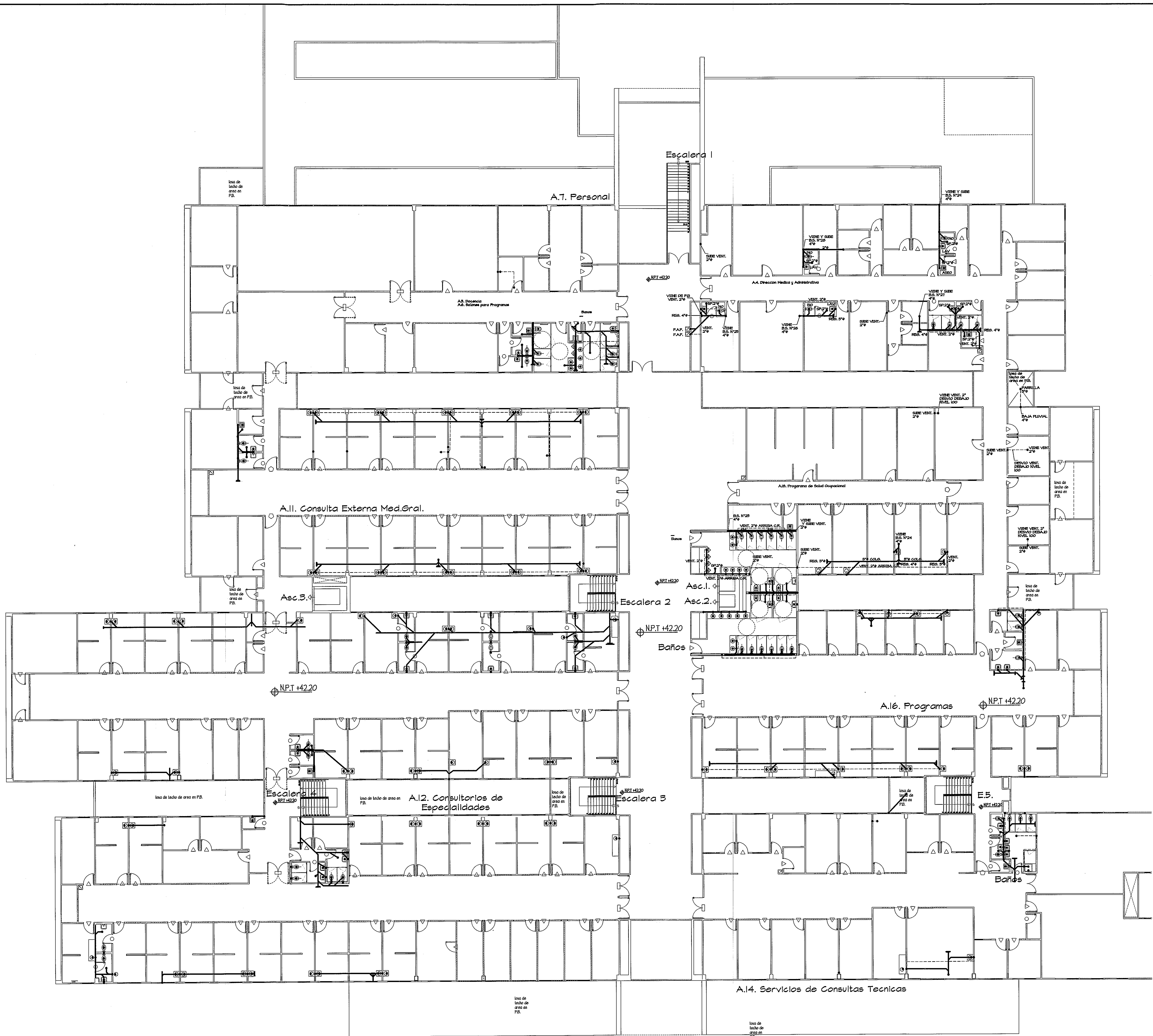
PLANTA GENERAL DE SISTEMA SANITARIO NIVEL 100 ESCALA 1:150 PLANTA NIVEL 100
