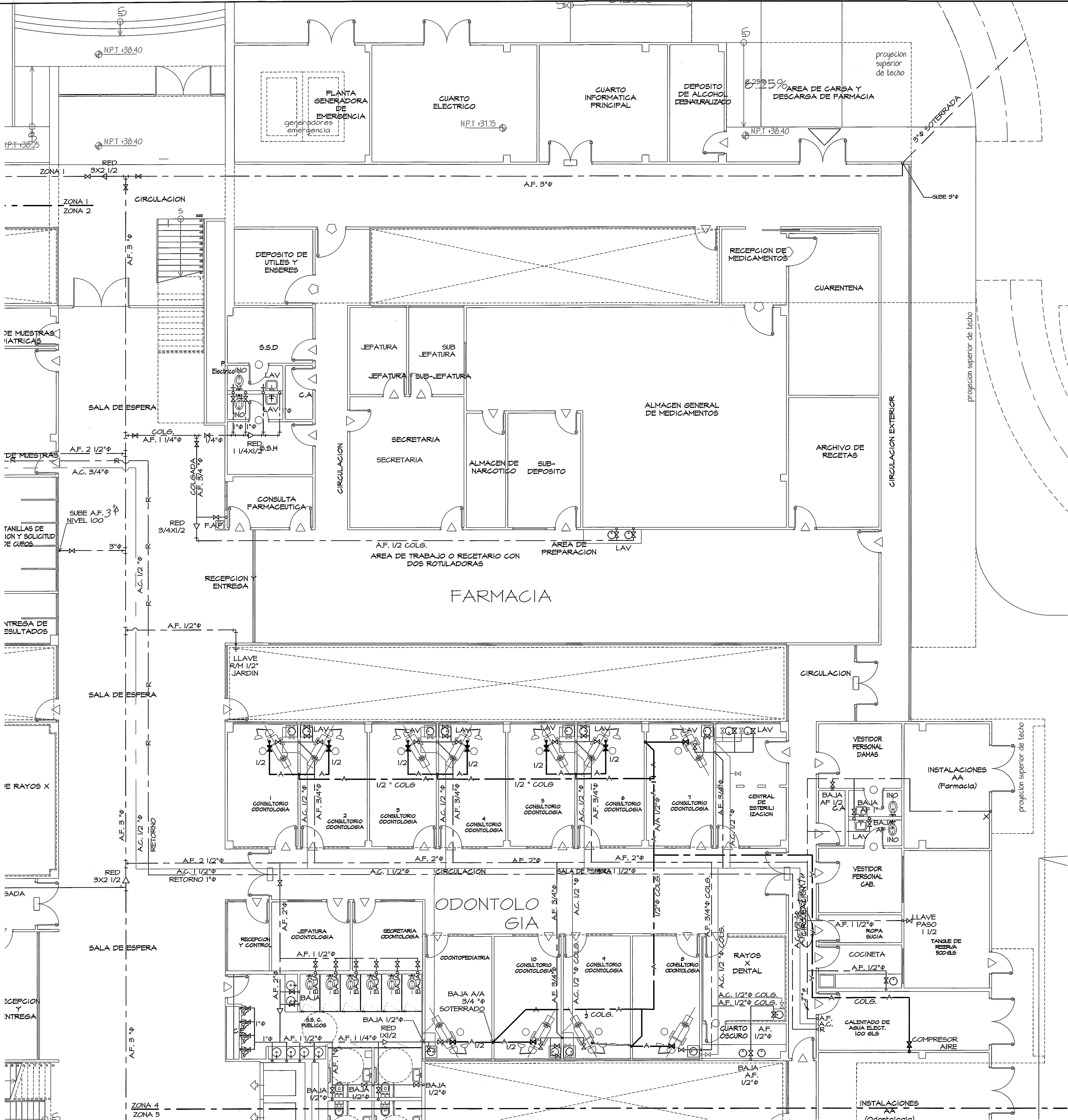
PLANTA AMPLIACION ZONA 4 SISTEMA AGUA POTABLE - NIVEL 000 ESCALA 1:75
