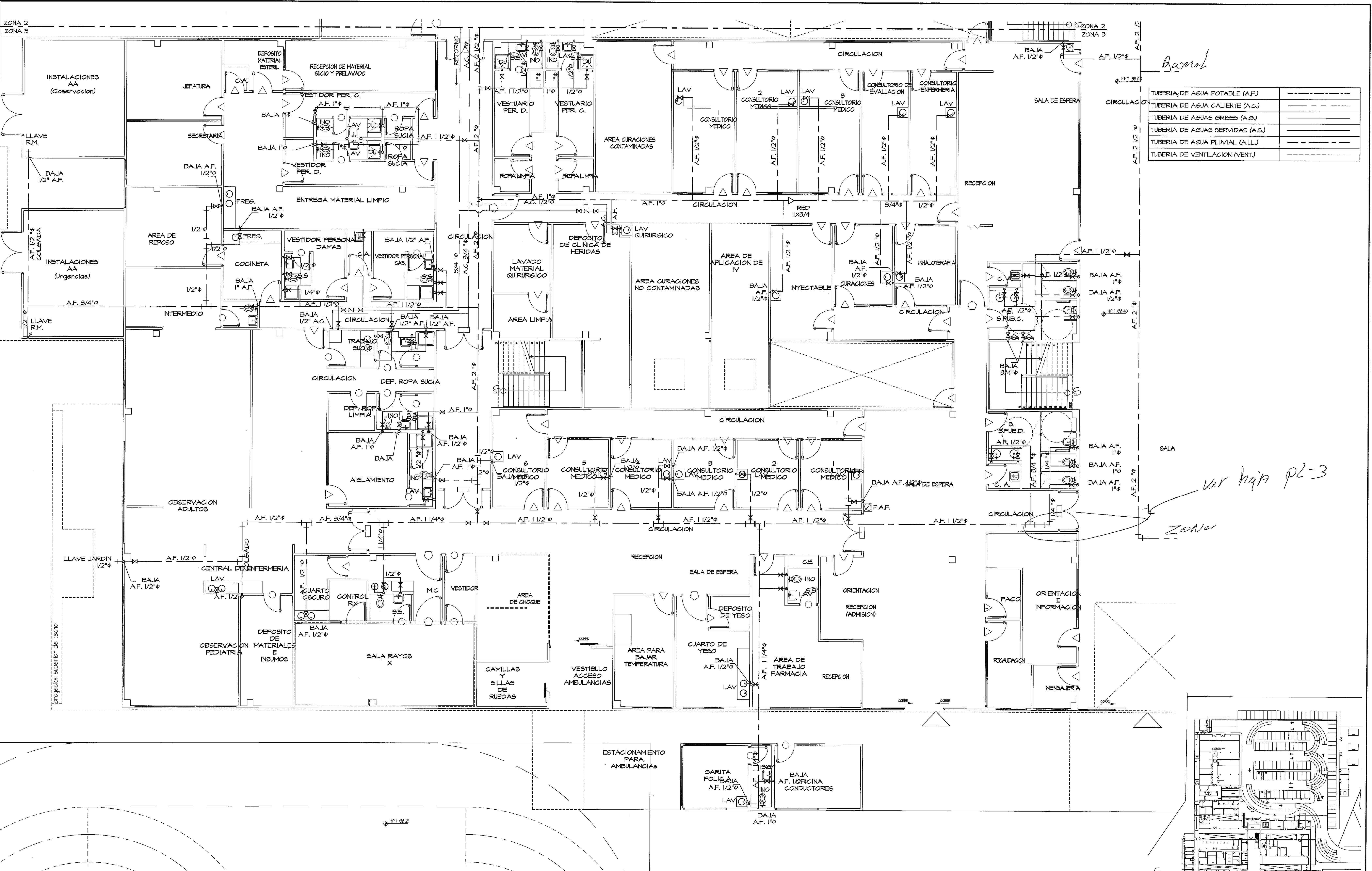
PLANTA AMPLIACION ZONA 3 SISTEMA AGUA POTABLE - NIVEL 000 ESCALA 1:75
