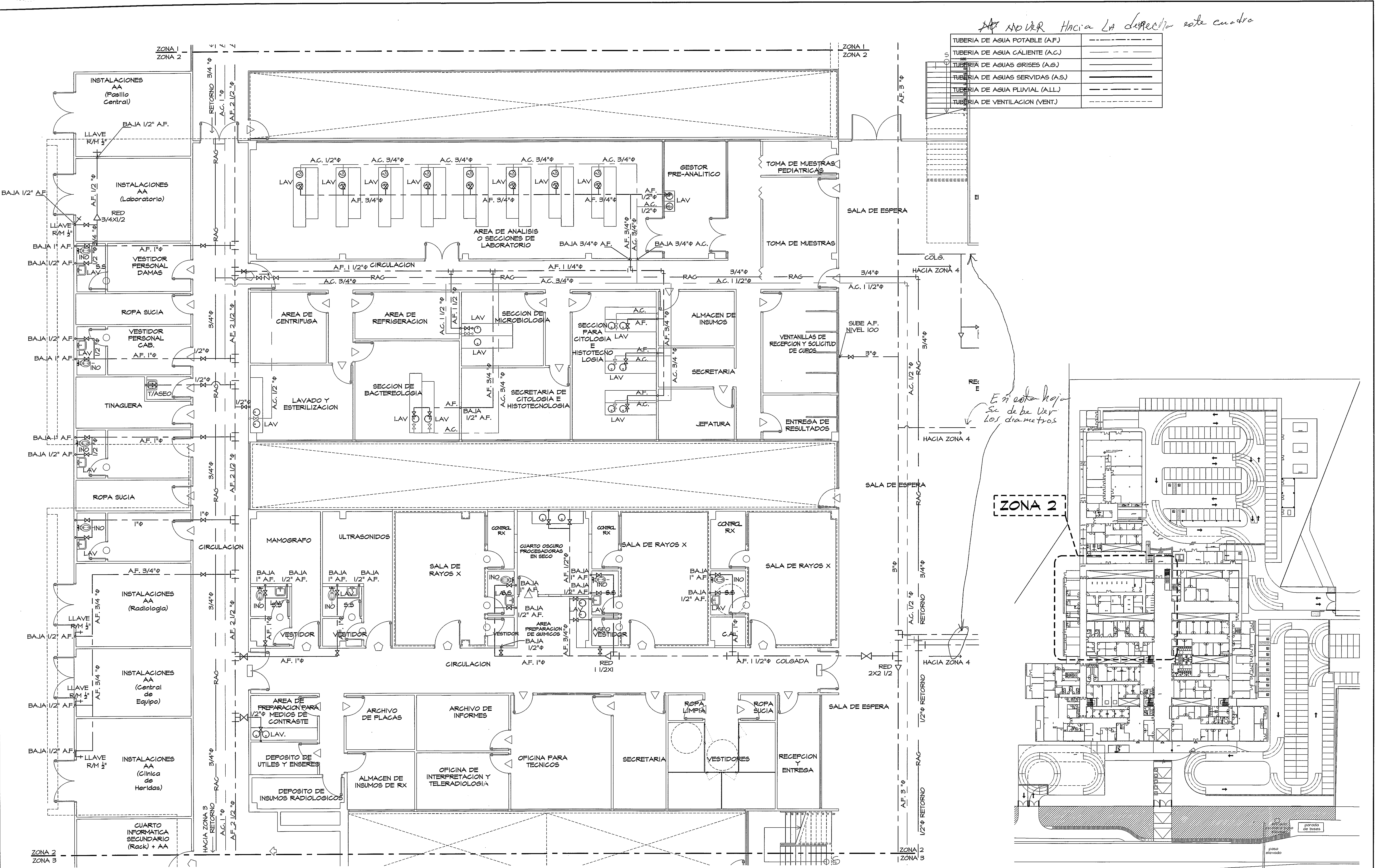
PLANTA AMPLIACION ZONA 2 SISTEMA AGUA POTABLE - NIVEL 000 ESCALA 1:75
