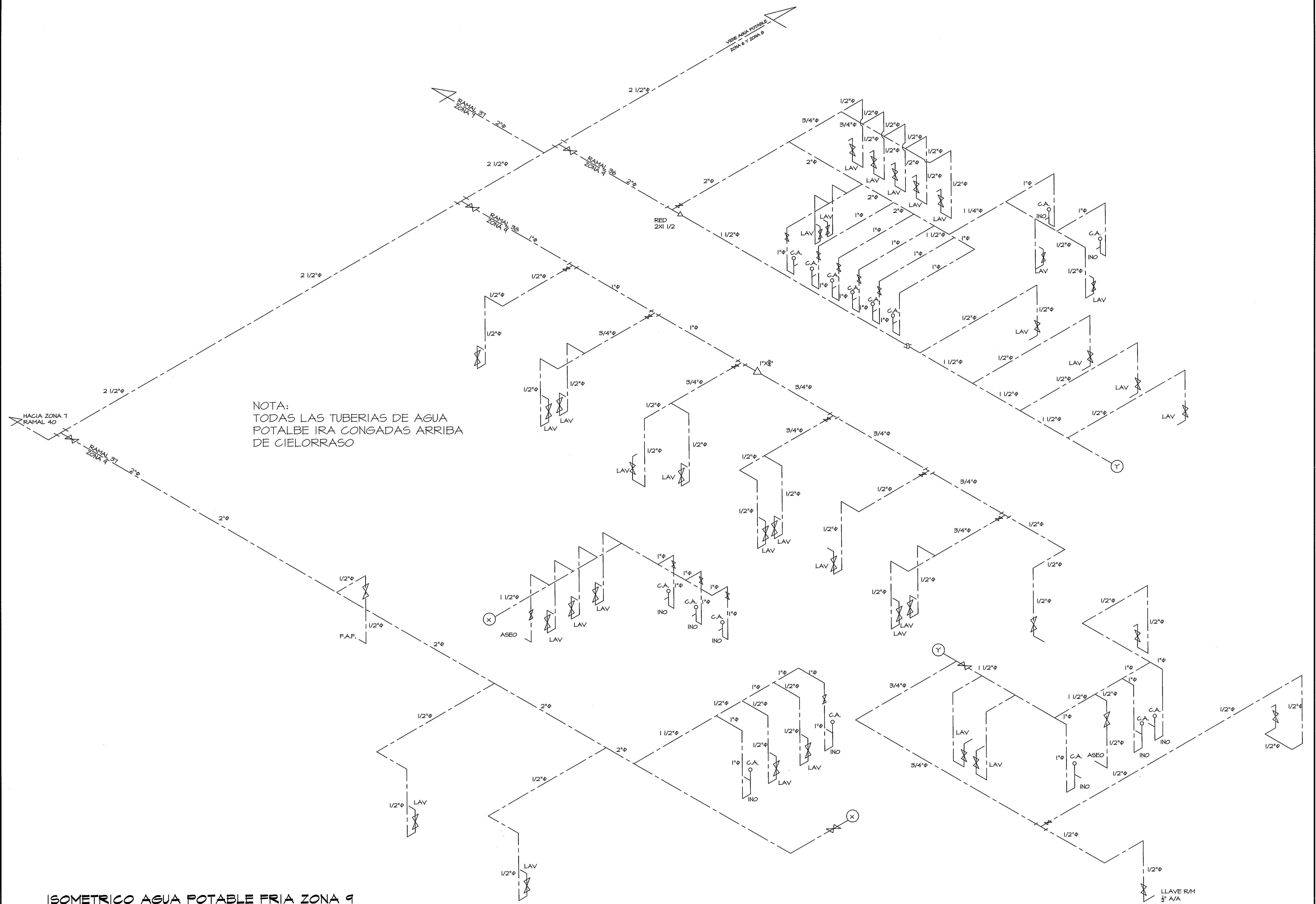
ISOMETRICO AGUA POTABLE FRIA ZONA 9 SIN ESCALA
