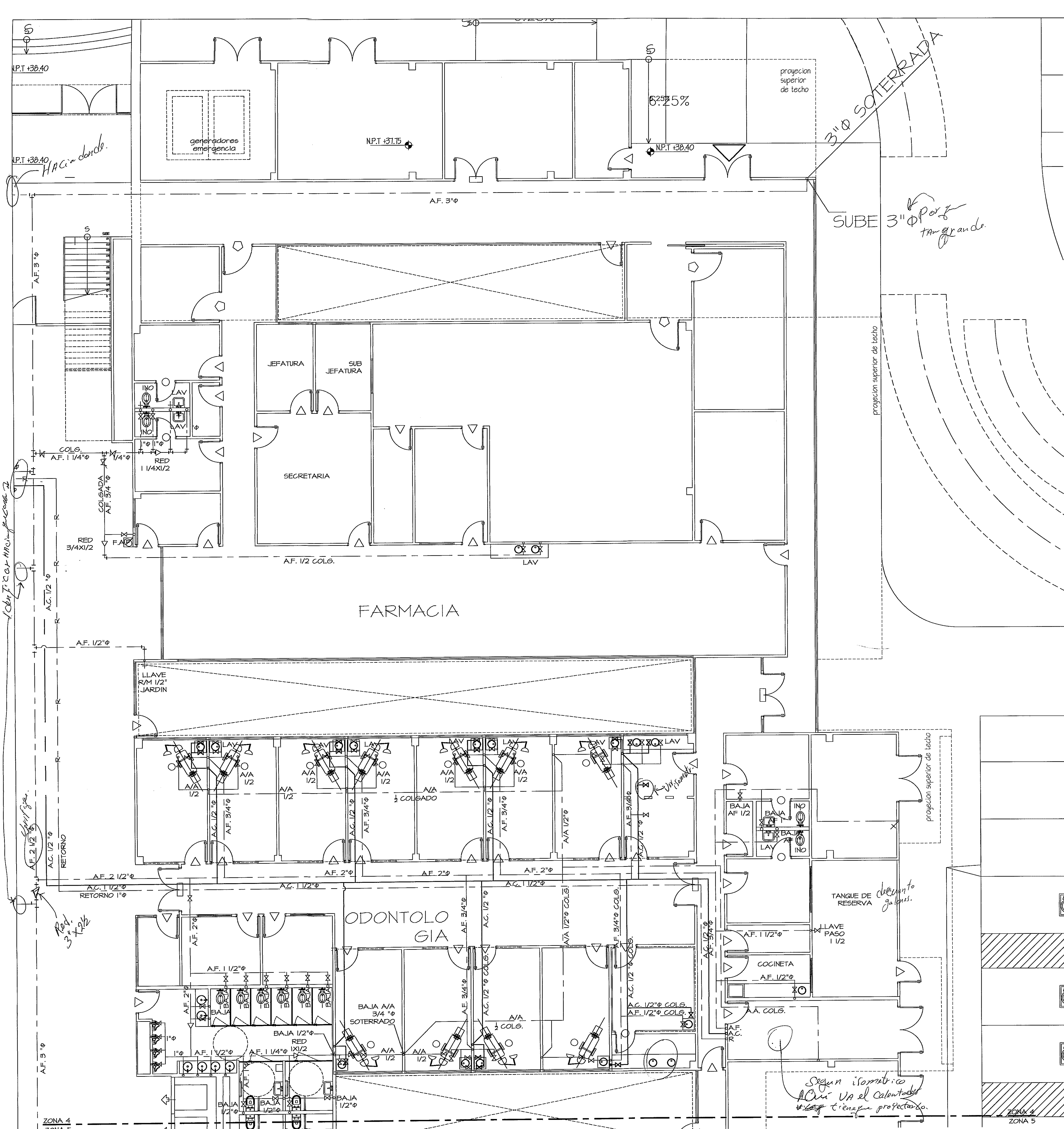
PLANTA AMPLIACION ZONA 4 SISTEMA AGUA POTABLE ESCALA 1:600
