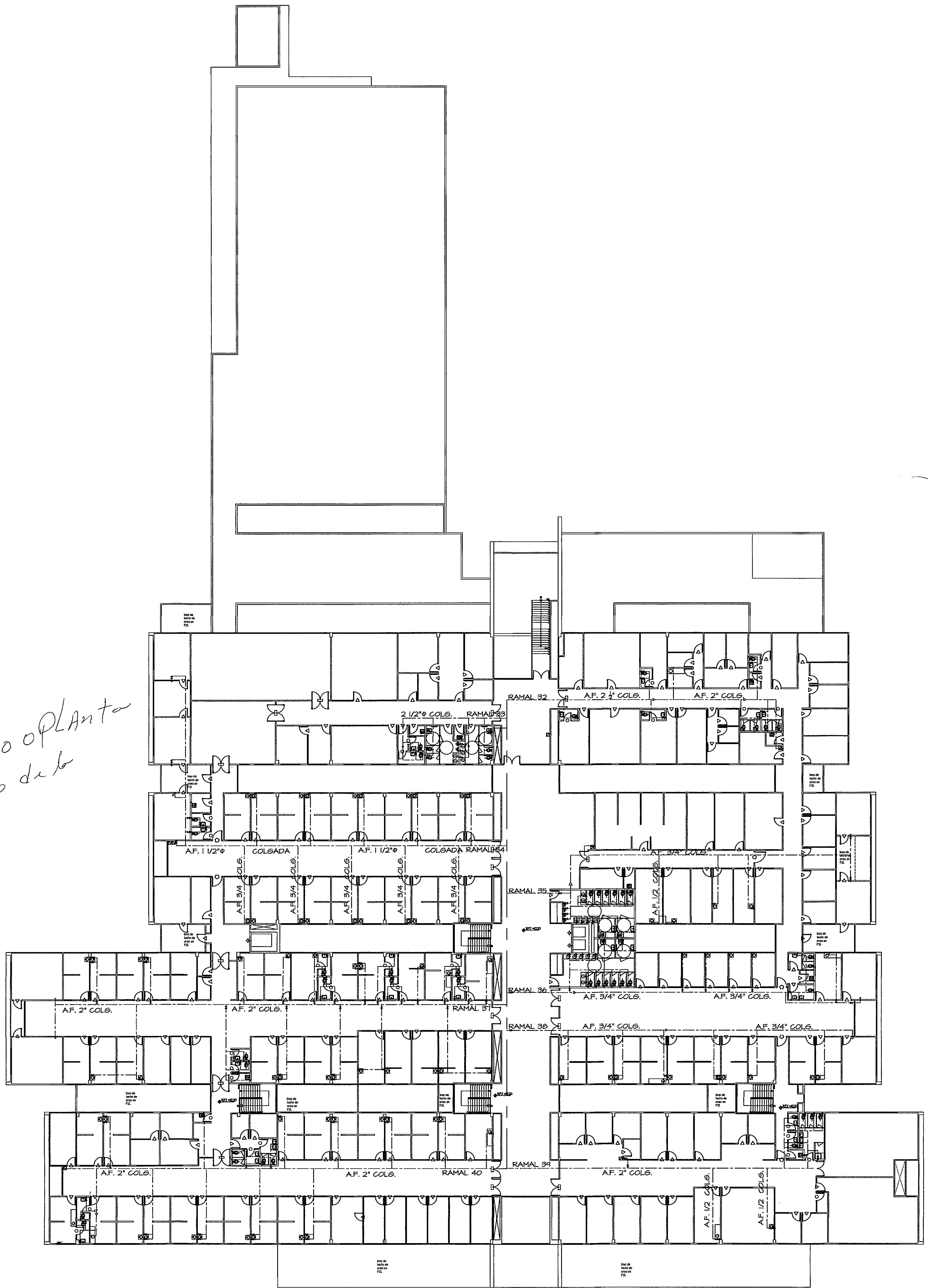
PLANTA GENERAL DE SISTEMA DE AGUA POTABLE (NIVEL 100) ESCALA 1:250
