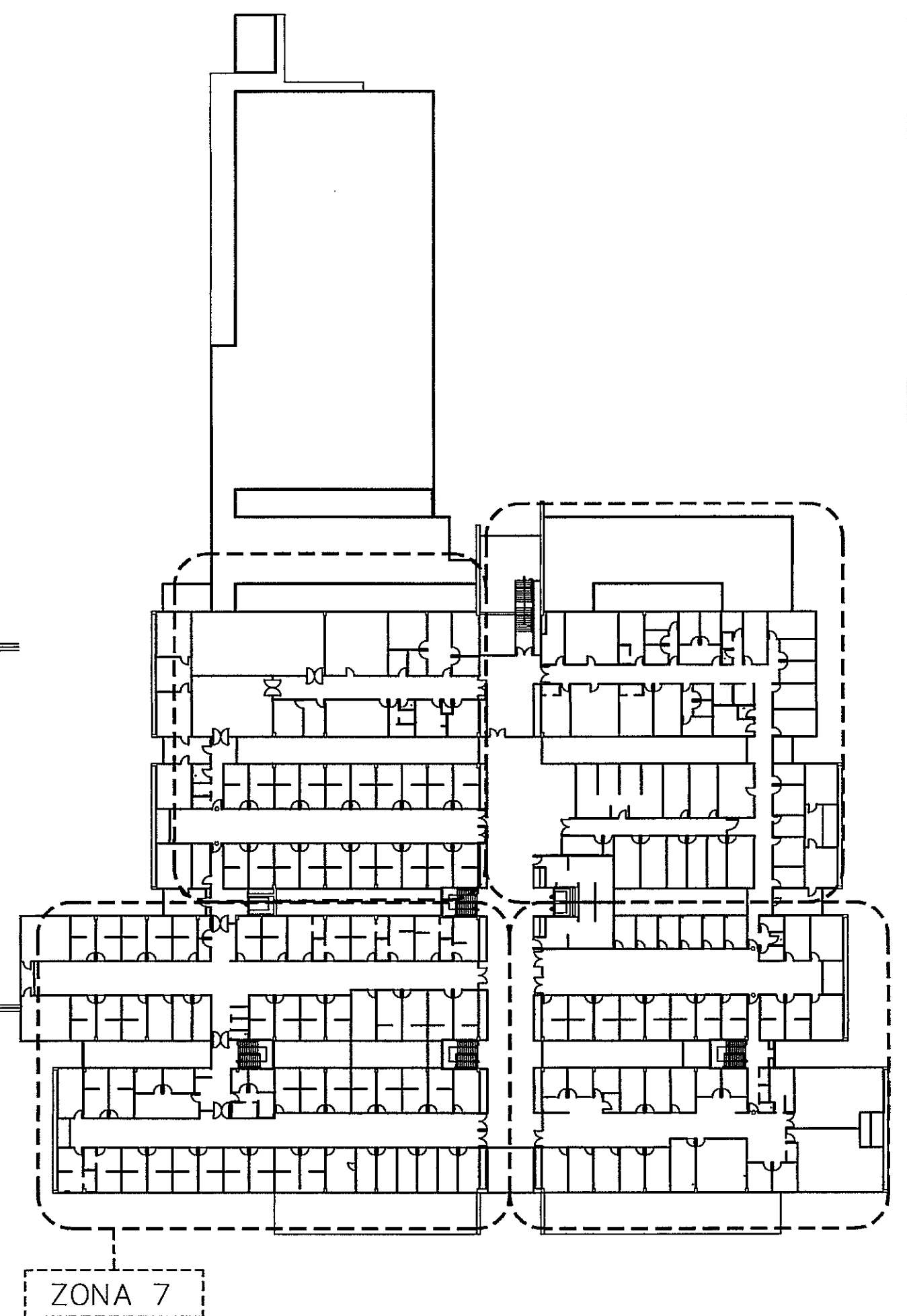
GUIA DE AMPLIACIONES POR ZONAS ESCALA - 1/500 / PLANTA ALTA (NIVEL 100)
