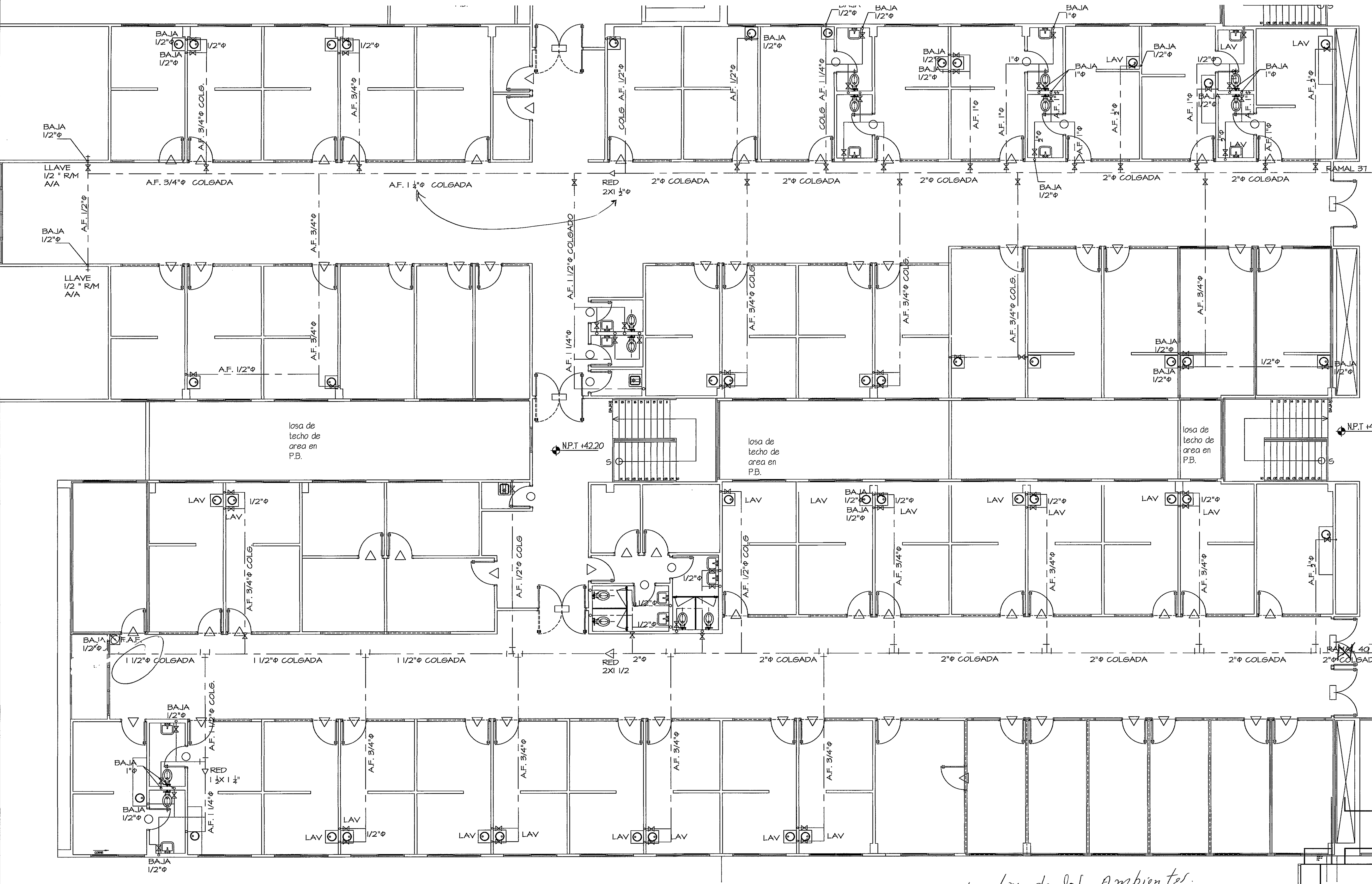
PLANTA AMPLIADA ZONA 7 SISTEMA DE AGUA POTABLE ESCALA 1:75
