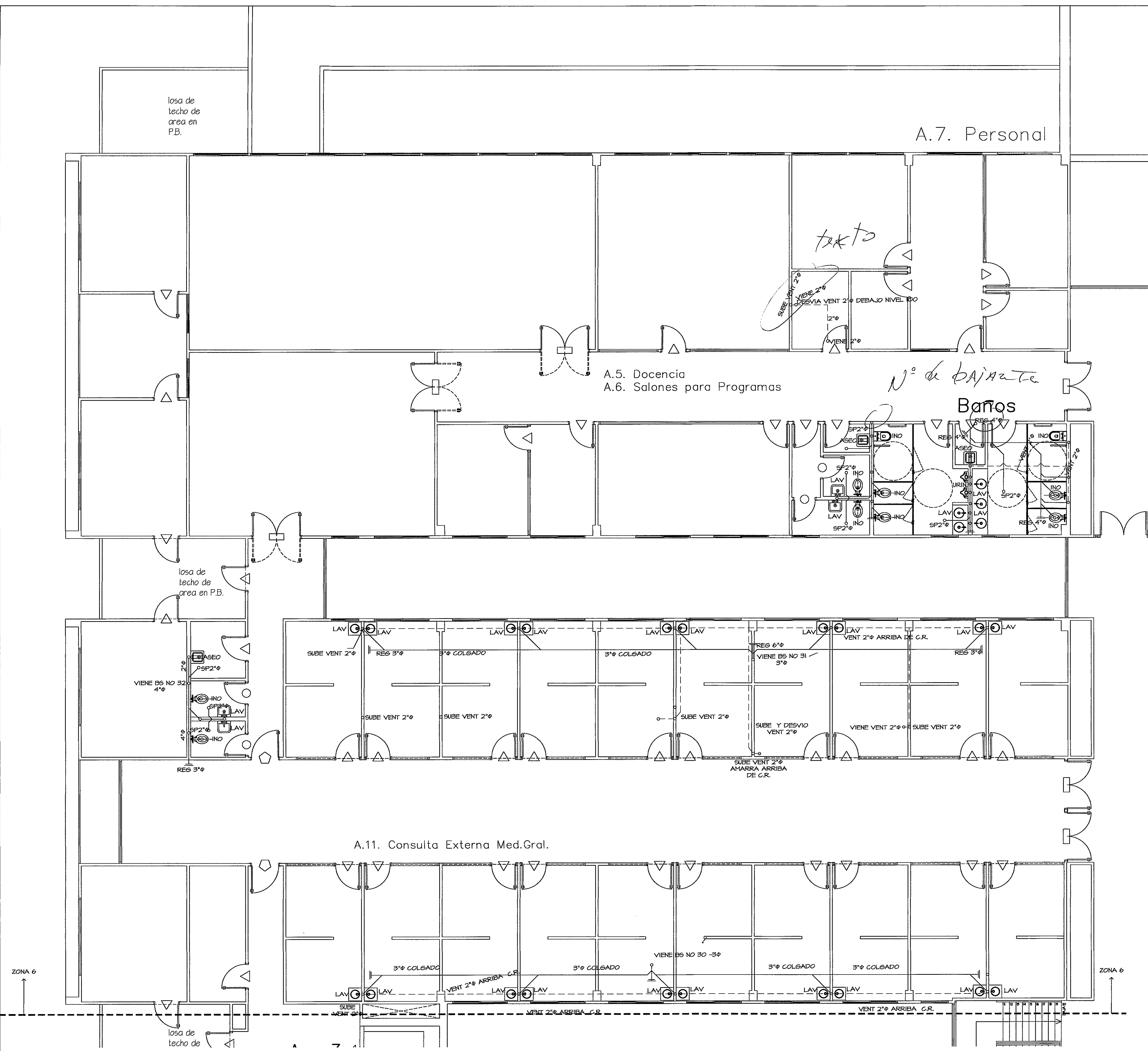
PLANTA AMPLIACION ZONA 6 SANITARIA Y PLUVIAL ESCALA 1:75
