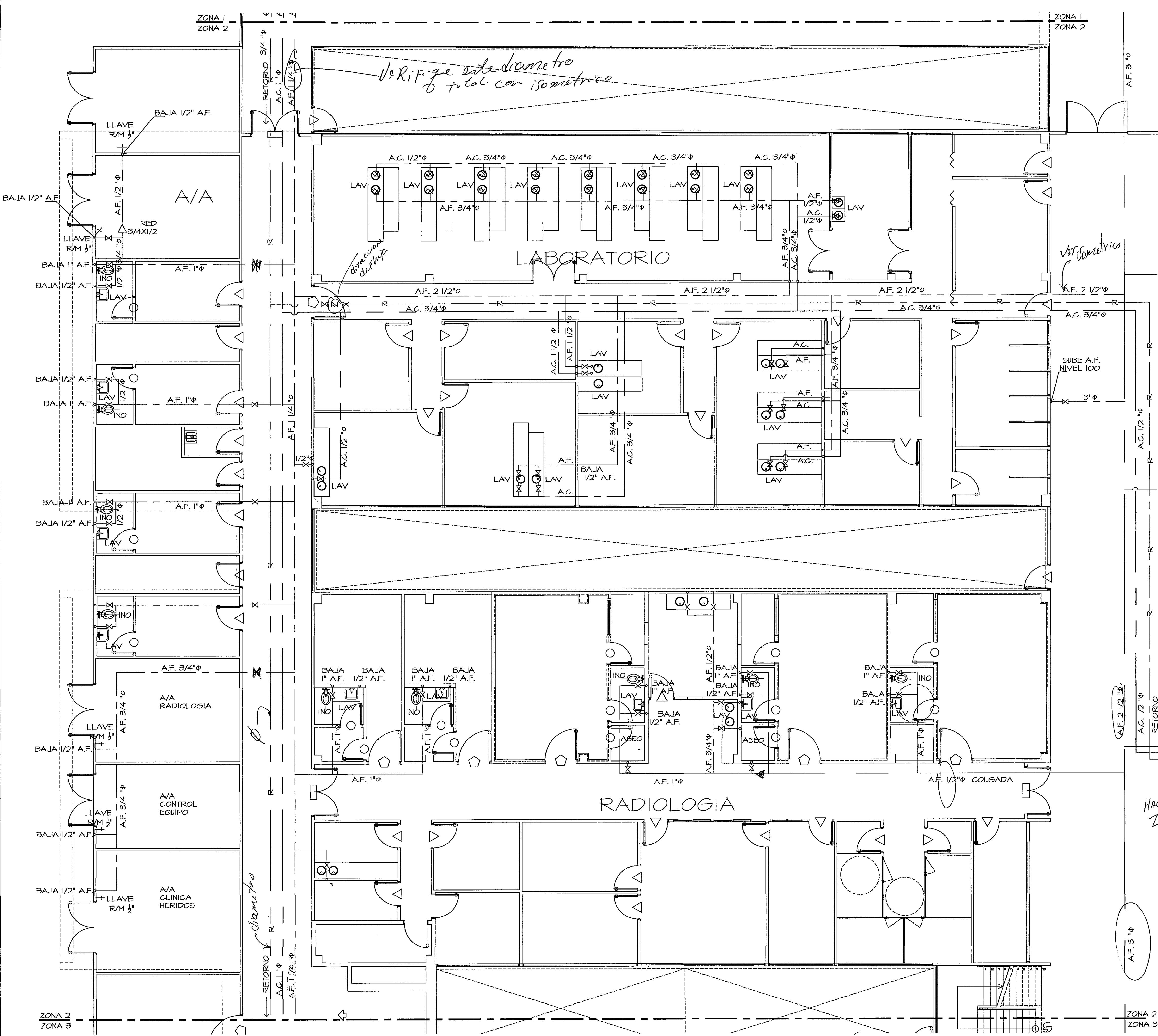
PLANTA AMPLIACION ZONA 2 SISTEMA AGUA POTABLE ESCALA 1:600
