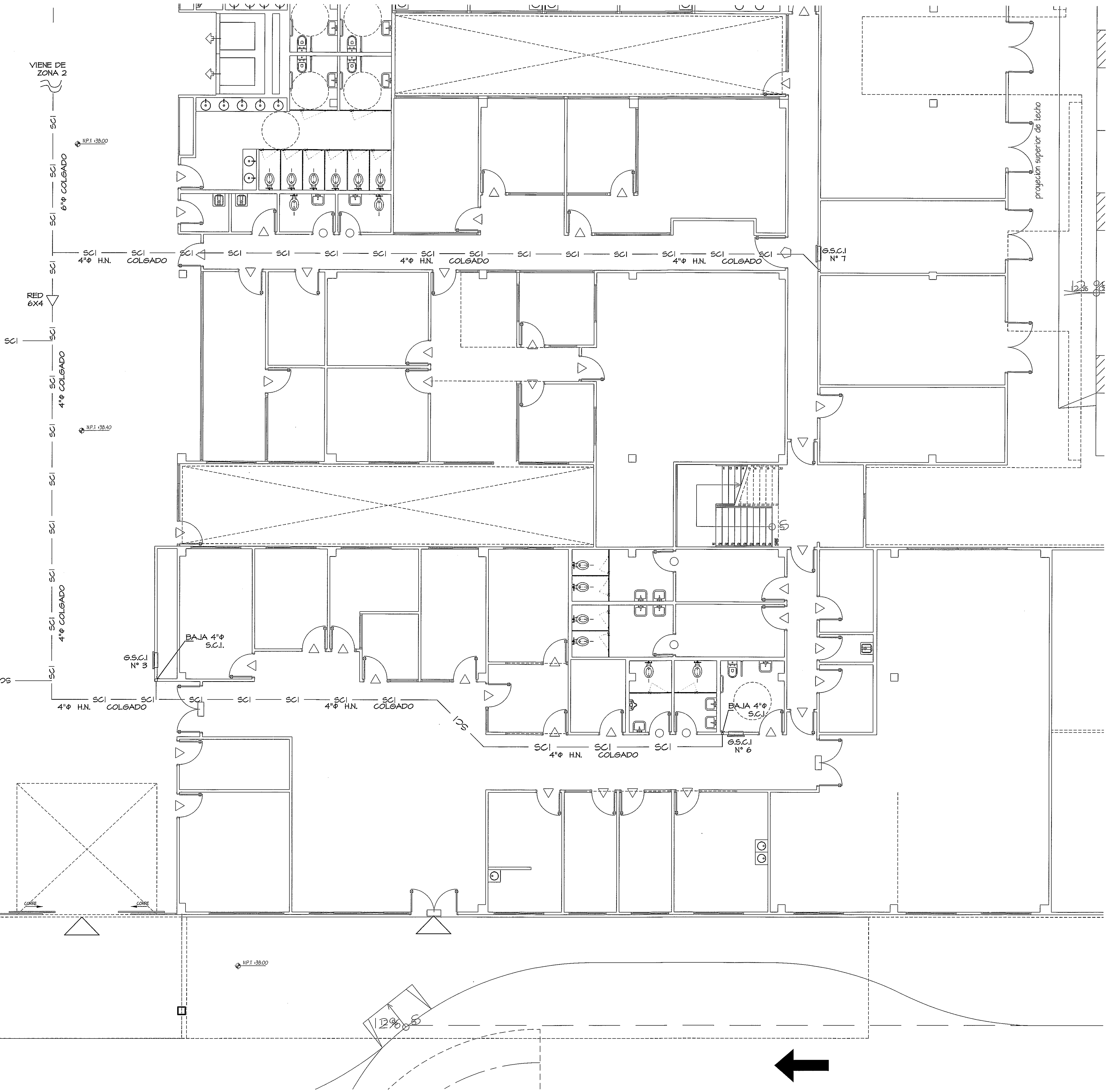
PLANTA AMPLIACION DE ZONA 5 SISTEMA CONTRA INCENDIO ESCALA 1:75
