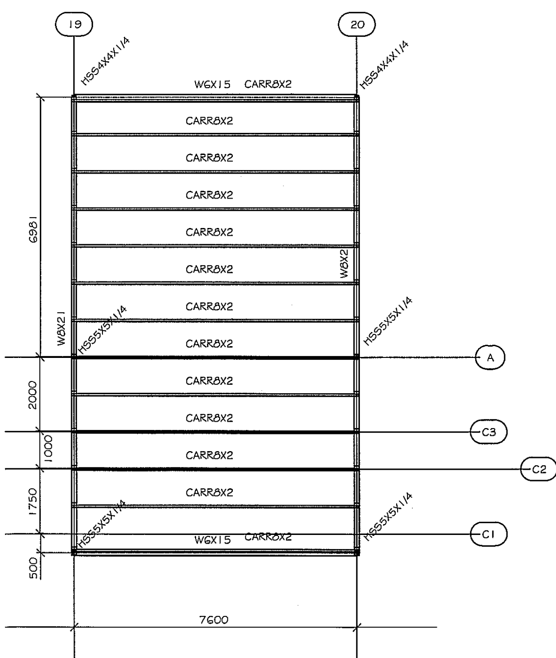
PLANTA - TECHO 3 ESCALA 1:100
