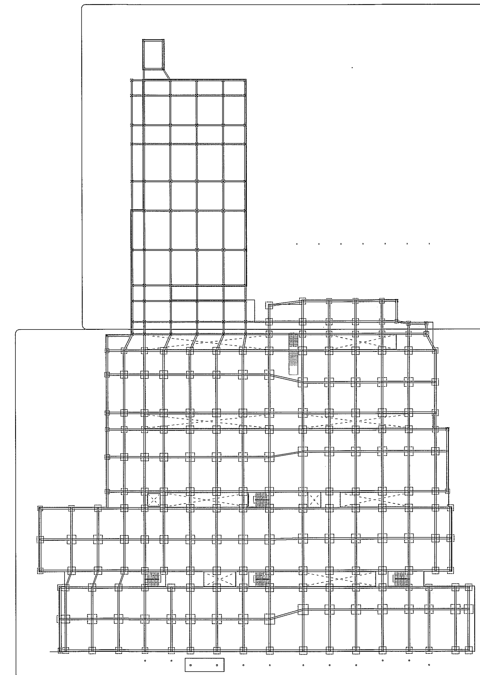
GUIA DE AMPLIACION POR ZONAS ESCALA 1:500
