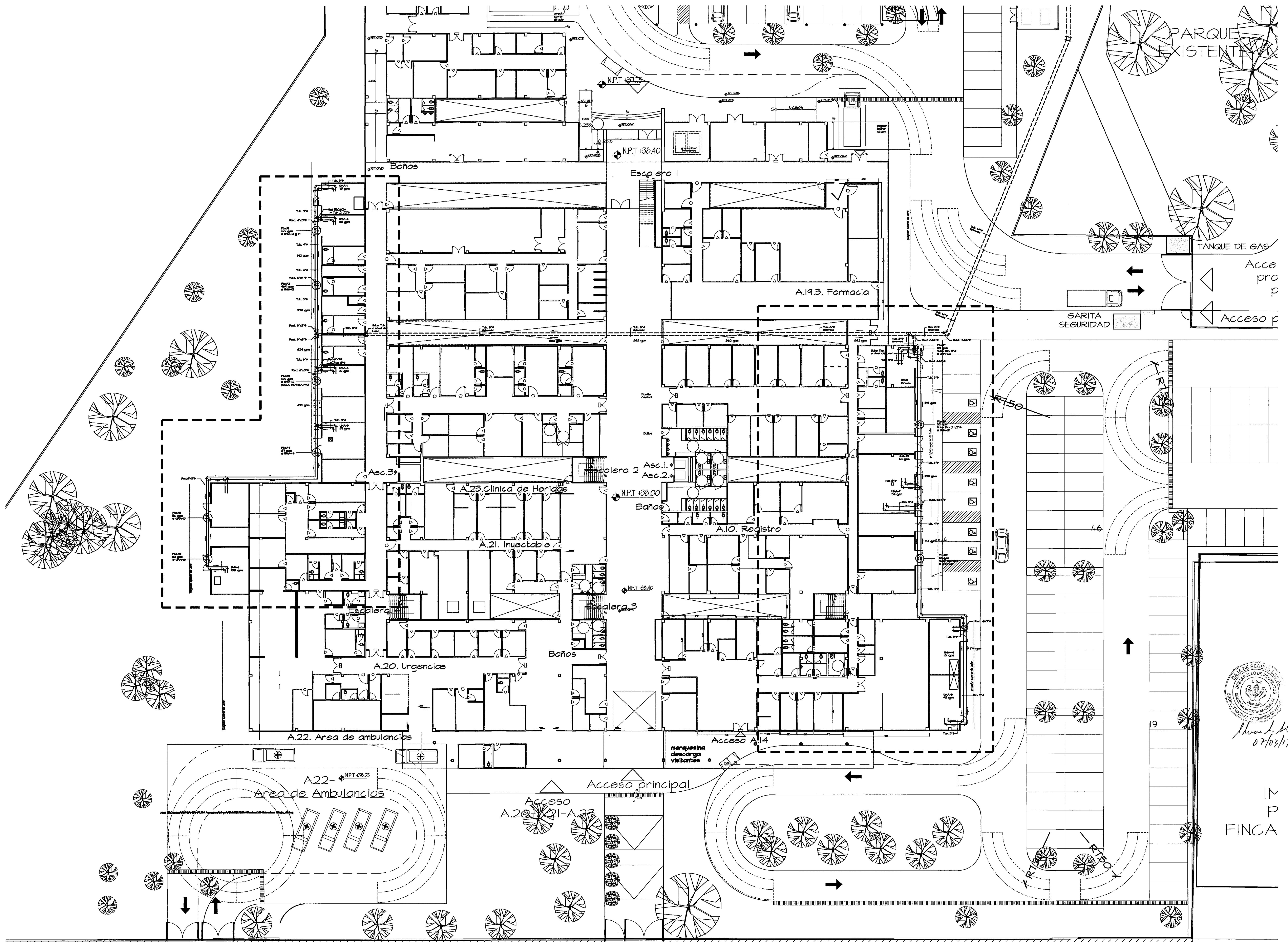
PLANTA BAJA TUBERIAS DE AGUA FRIA GENERAL ESCALA.- 1/200
