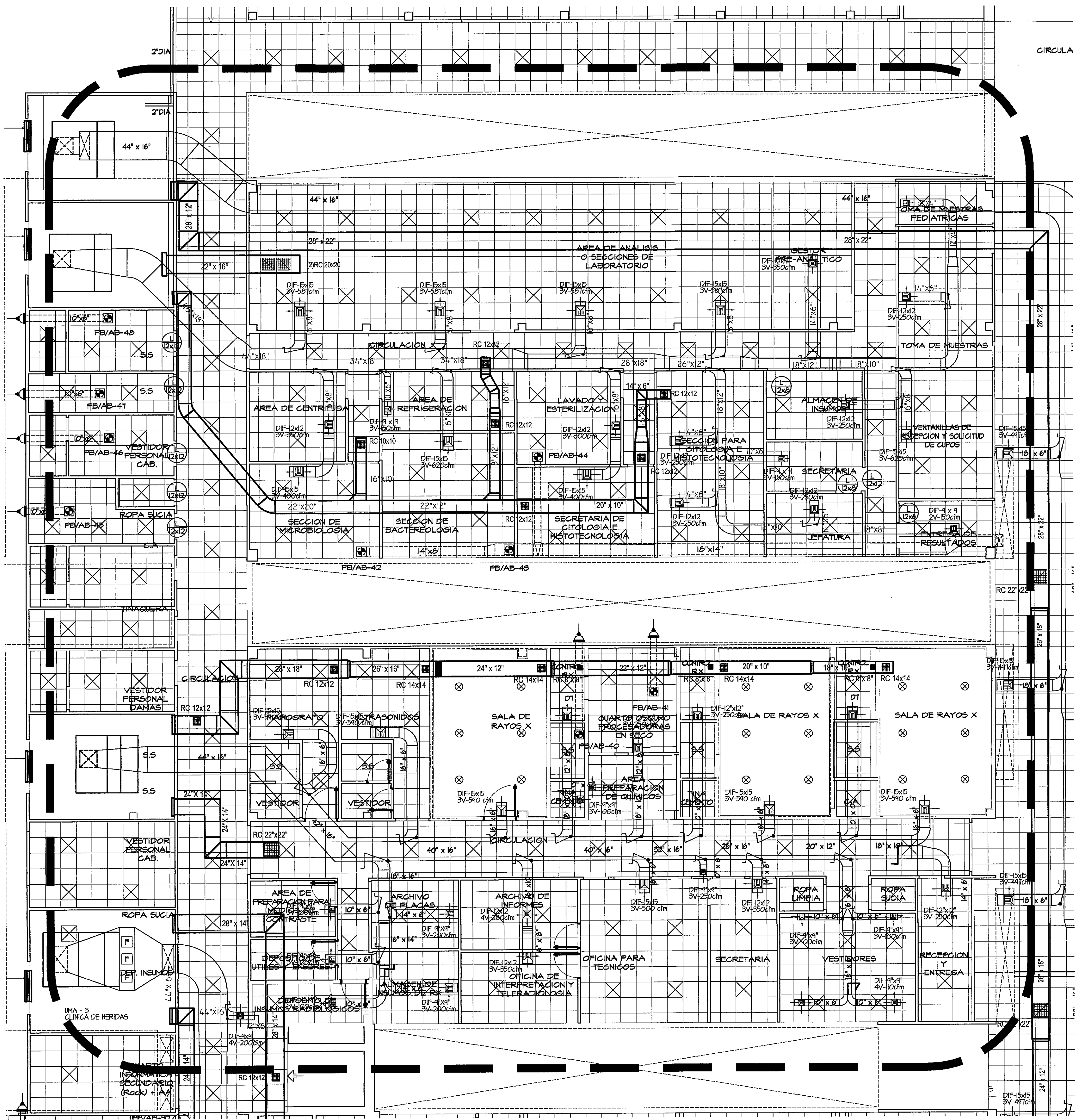
PLANTA DE AIRE ACONDICIONADO-ZONA #2 PLANTA BAJA ESCALA.- 1/75
