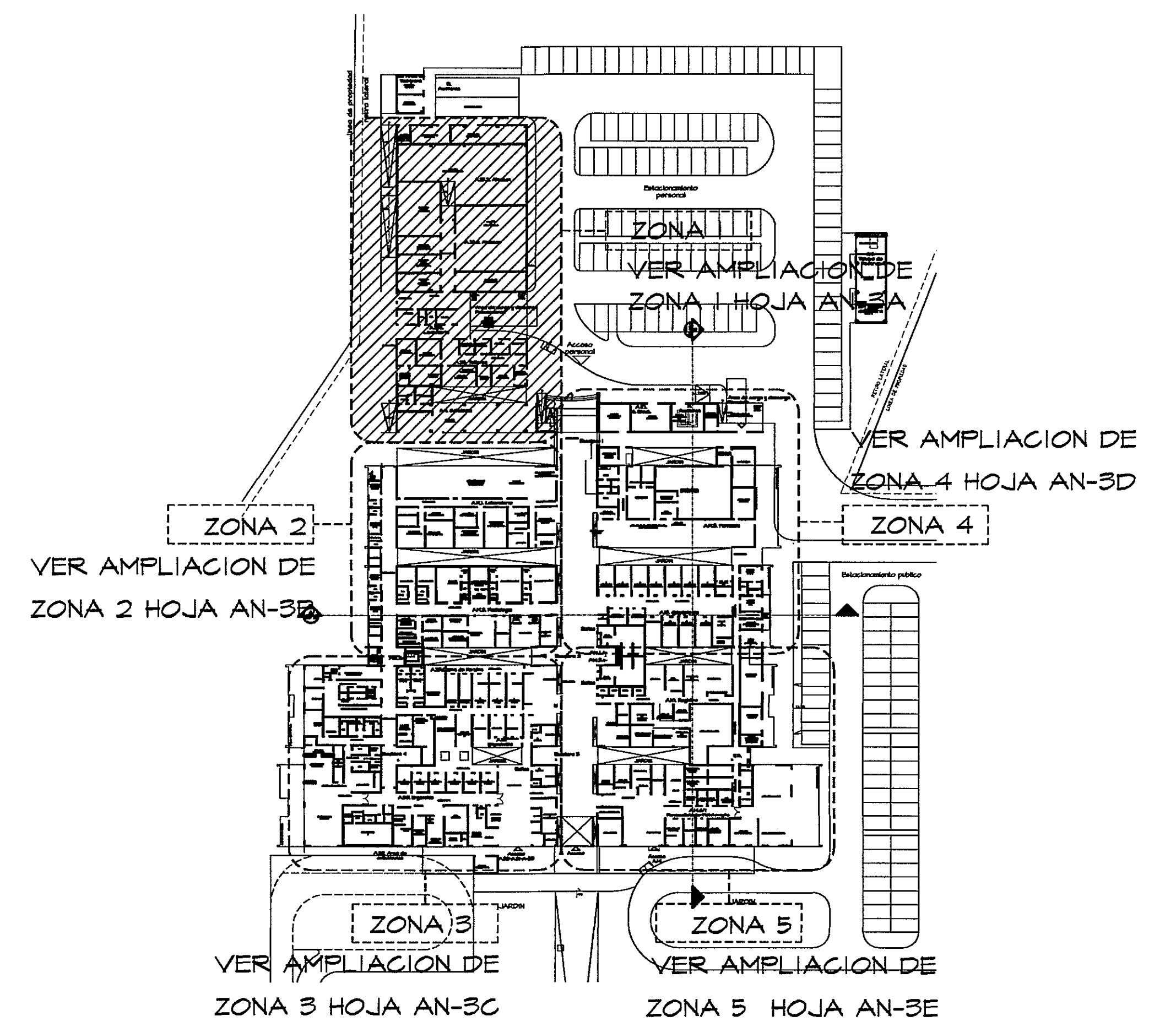
GUIA DE AMPLIACIONES POR ZONAS ESCALA.- 1/750 PLANTA BAJA (NIVEL 000, -050, -100)
