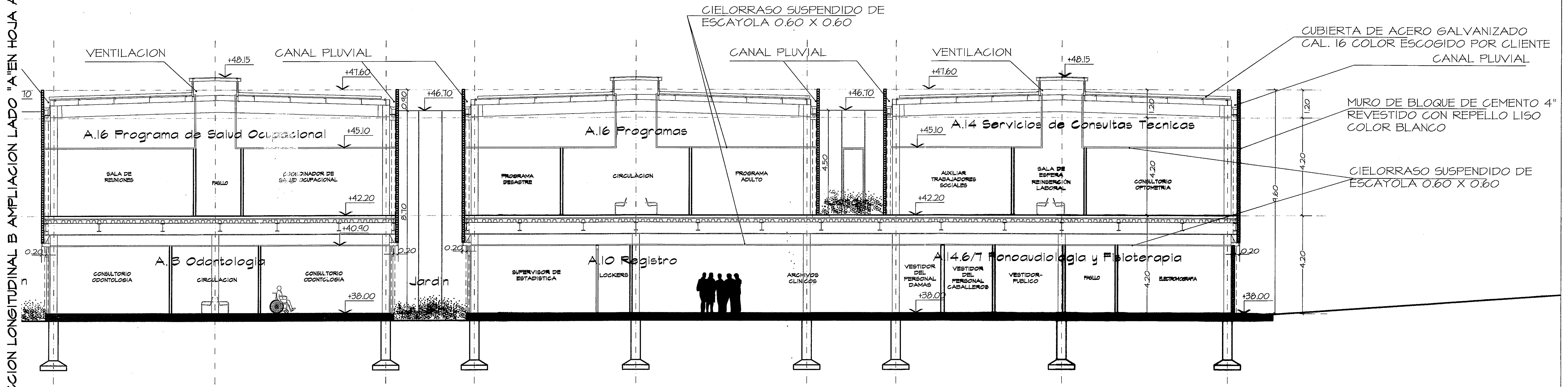
SECCION LONGITUDINAL B ampliacion lado B ESC. 1:75
