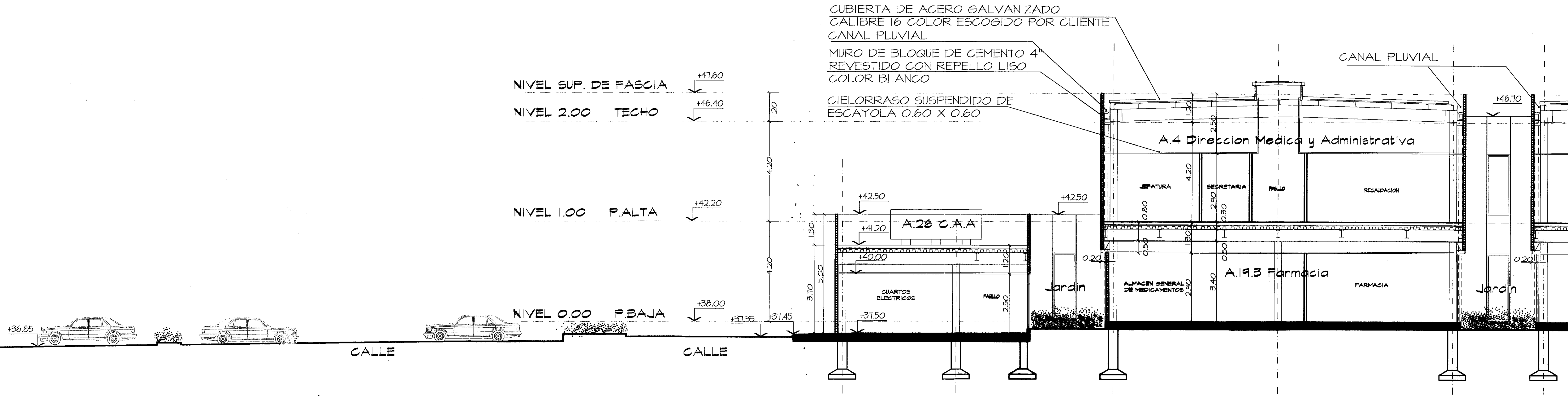
SECCION LONGITUDINAL B ampliacion lado A ESC. 1:75
