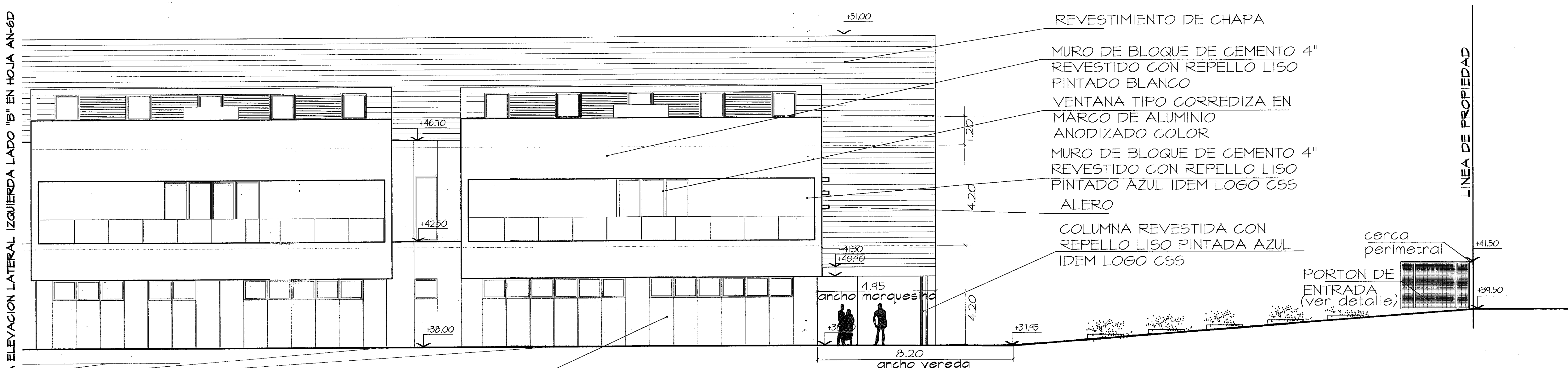
ELEVACION LATERAL IZQUIERDA - AMPLIACION LADO "C" ESC.1:75
