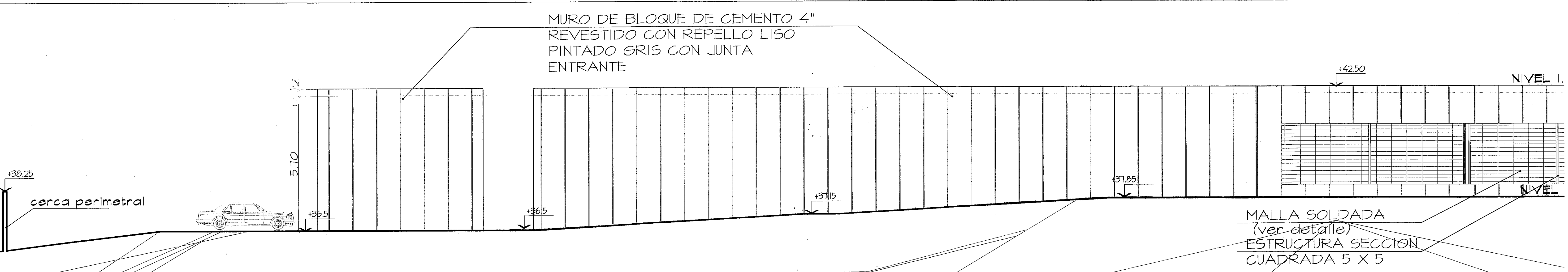
ELEVACION LATERAL IZQUIERDA - AMPLIACION LADO "A" ESC.1:75
