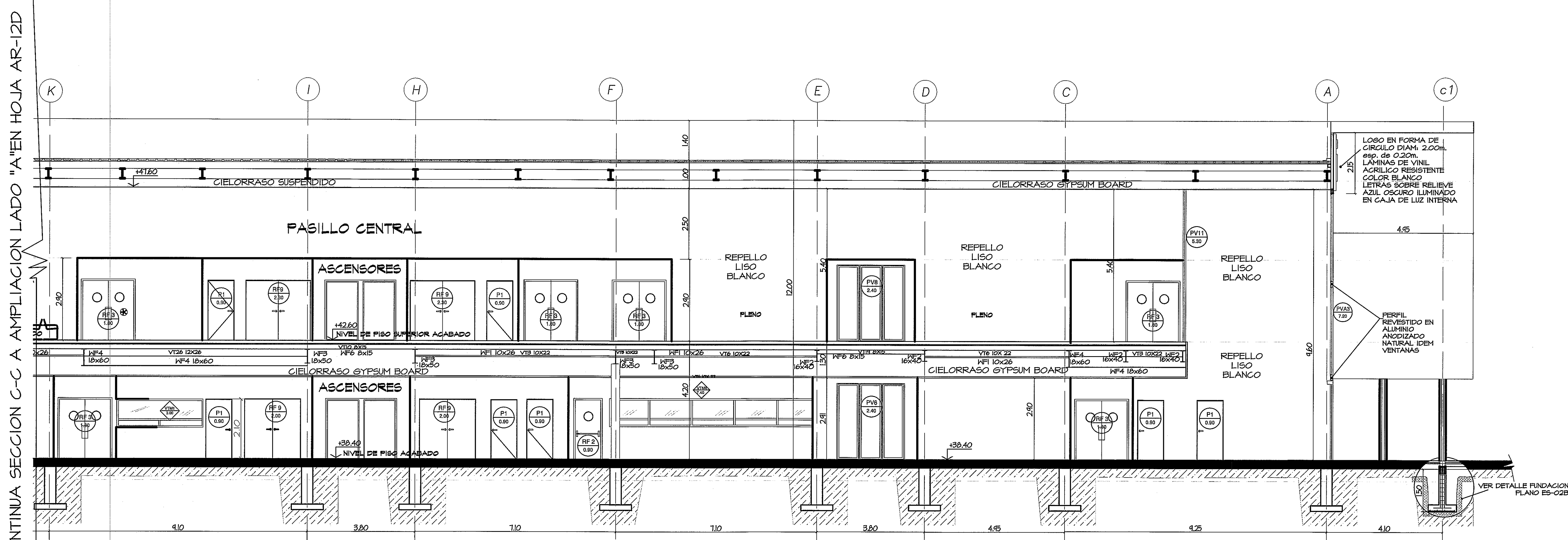
SECCION C-C ampliacion lado A esc 1:75
