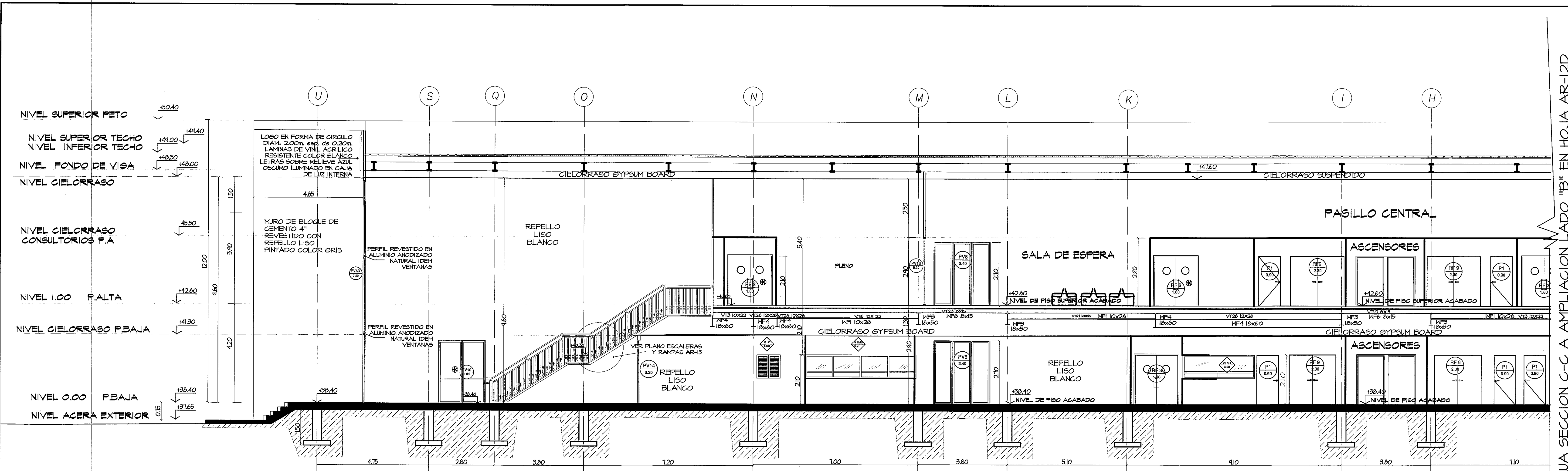
SECCION C-C ampliacion lado A esc 1:75
